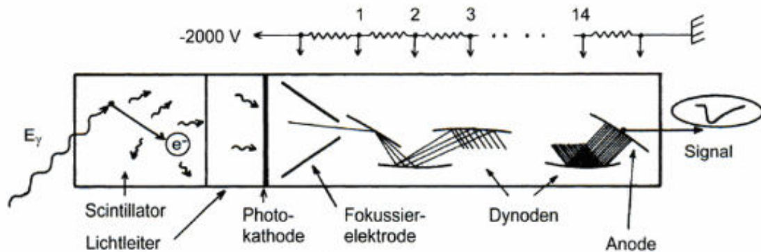
Abbildung 12: Schematischer Aufbau eines NaI-Detektors [82].
