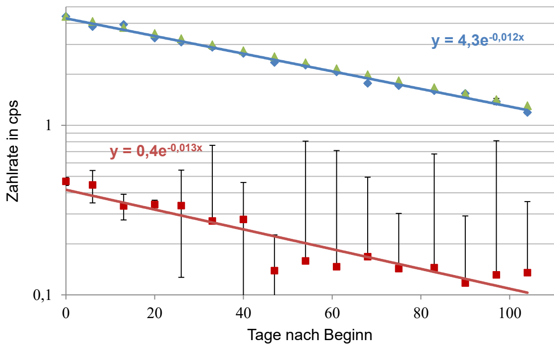
Abbildung 53: Zählraten Glas 4, synthetisches Meerwasser mit Benzoat-, Toluol-, Glucose- und ^{125}\text{I}^- -Zugabe. pH = 7,7 und Eh = 414,7 mV. \blacklozenge ^{125}\text{IO}_3^- , \blacksquare ^{125}\text{I}^- , \blacktriangle ^{125}\text{I}^- rechnerisch.
