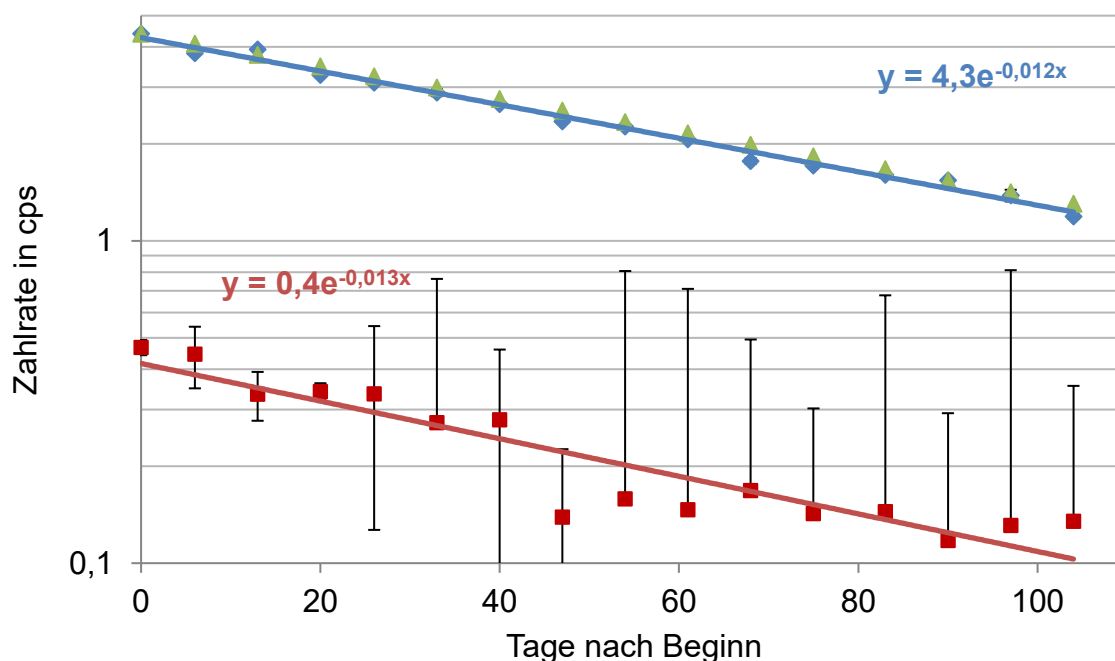
Abbildung 67: Zählraten aus dem Glas 5 des zweiten Batch Experimentes. Synthetisches Meerwasser mit ^{125}\text{I O}_3^- -Zugabe. pH = 8,2 und Eh = 401,5 mV. \blacklozenge ^{125}\text{I O}_3^- , \blacksquare ^{125}\text{I}^- , \blacktriangle ^{125}\text{I O}_3^- rechnerisch.
