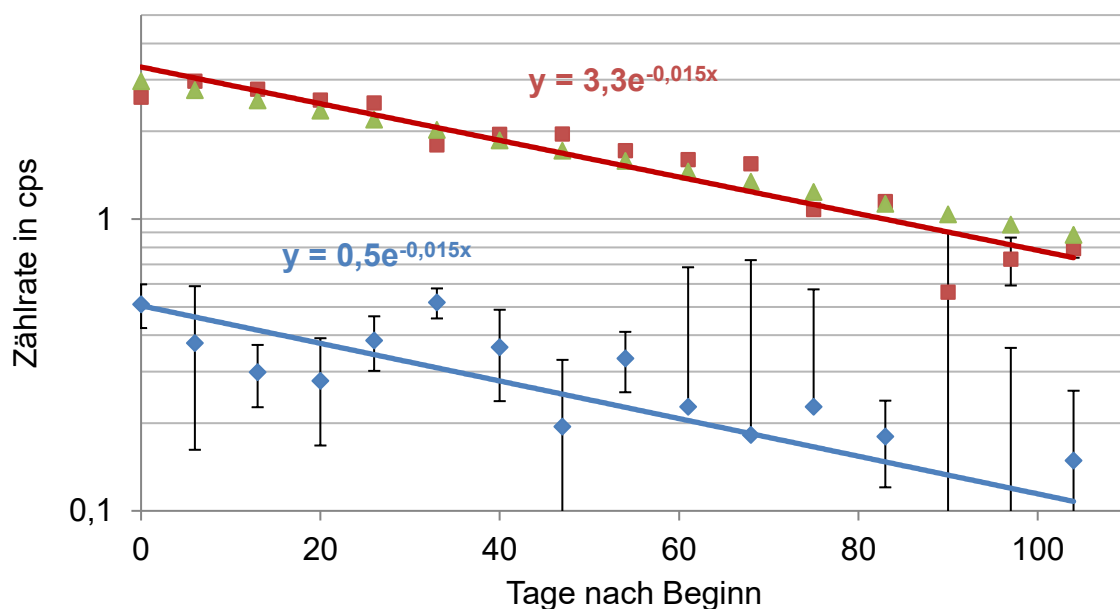
Abbildung 65: Messwerte aus dem Glas 1 des zweiten Batch Experimentes. Synthetisches Meerwasser mit ^{125}\text{I}^- -Zugabe. pH = 7,4 und Eh = 464,1 mV. \diamond ^{125}\text{IO}_3^- , \blacksquare ^{125}\text{I}^- , \blacktriangle ^{125}\text{I}^- rechnerisch.
