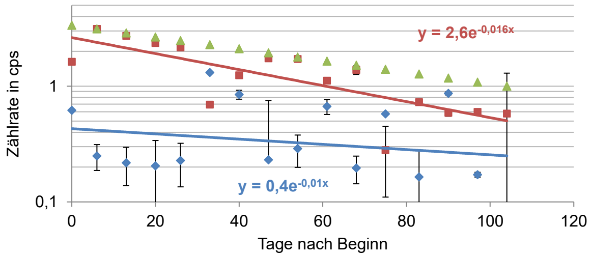
Abbildung 65: Messwerte aus dem Glas 1 des zweiten Batch Experimentes. Synthetisches Meerwasser mit ^{125}\text{I}^- -Zugabe. pH = 7,4 und Eh = 464,1 mV. \diamond ^{125}\text{IO}_3^- , \blacksquare ^{125}\text{I}^- , \blacktriangle ^{125}\text{I}^- rechnerisch.
