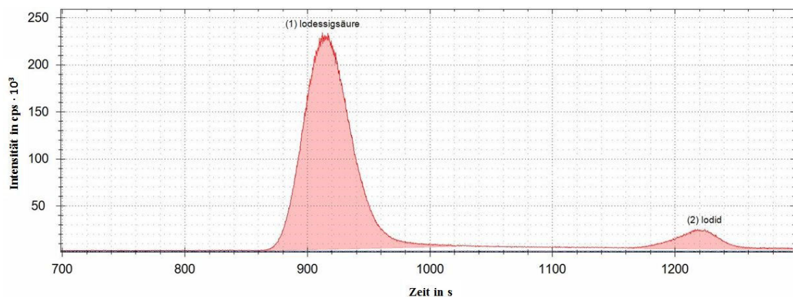
Abbildung 23: Chromatogramm einer lodessigsäurelösung mit [I] = 10 \mu\text{g}/\text{kg} .
