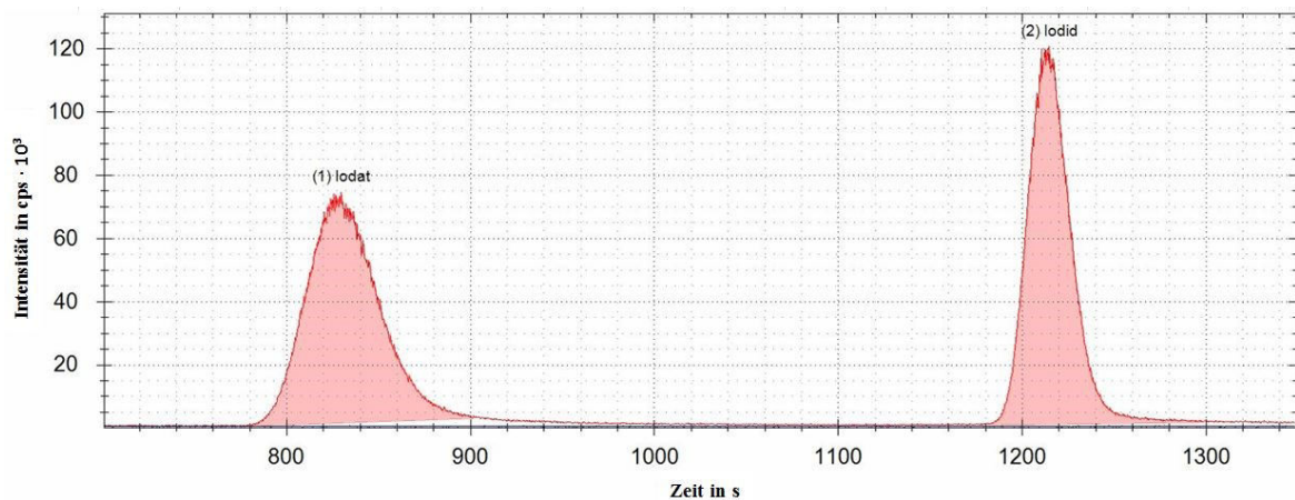
Abbildung 22: Chromatogramm einer Lösung mit lodat und lodid mit je [I] = 10 \mu\text{g}/\text{kg} .
