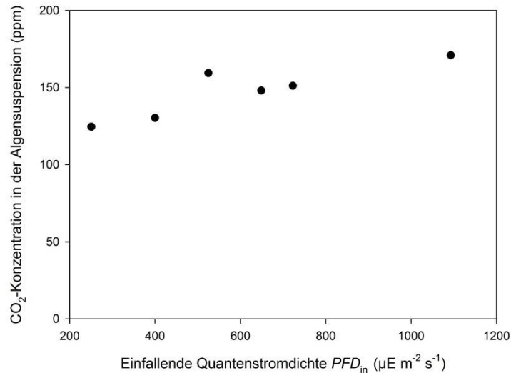
Abbildung 5-28: CO 2 -Konzentrationen der Kultursuspensionen an Tag 5 der Kurzzeit-Kultivierung verschiedener Versuchsvarianten bei unterschiedlichen Quantenstromdichten PFDI_{in} unter weißen LEDs
