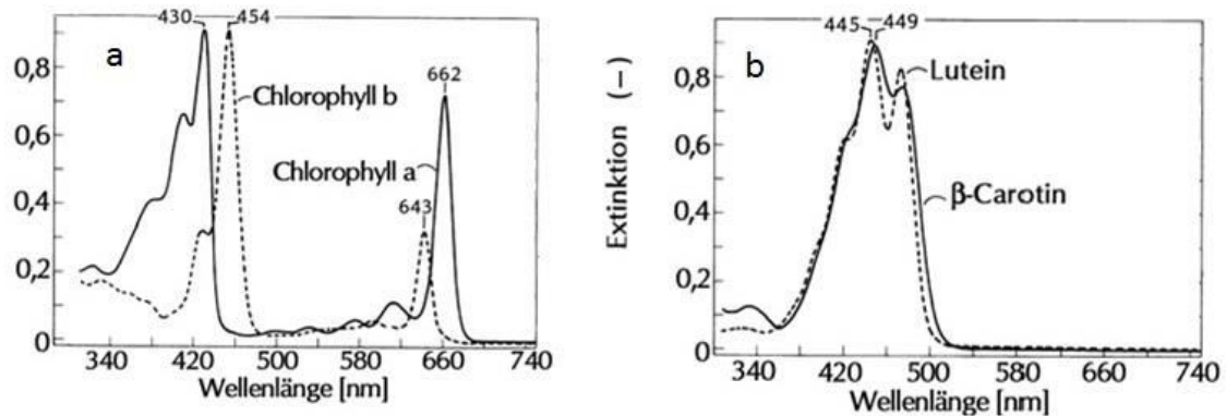
Abbildung 2-7: Relative Extinktionsspektren von Chl a und b und der Xanthophylle \beta -Carotin und Lutein über den Wellenlängenbereich von 300 nm – 740 nm in Diethylether. a: Chl a (durchgezogene Linie) und Chl b (gestrichelte Linie), b: \beta -Carotin (durchgezogene Linie) und Lutein (gestrichelte Linie) (verändert nach Schopfer & Brennicke 2010)
