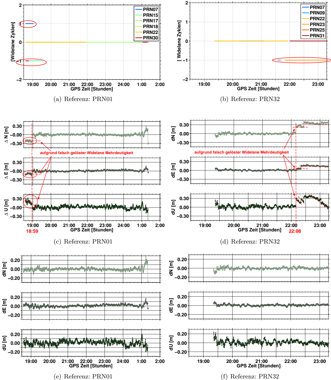
Abbildung 6.15: Beeinträchtigung der Widellane-Mehrdeutigkeitsanalyse und der Widellane-Koordinatenbestimmung durch GDV für zwei verschiedene Referenzsatelliten (a-d) sowie Korrektur der Koordinatenlösung durch Berücksichtigung der GDV-Korrekturen (e-f).
