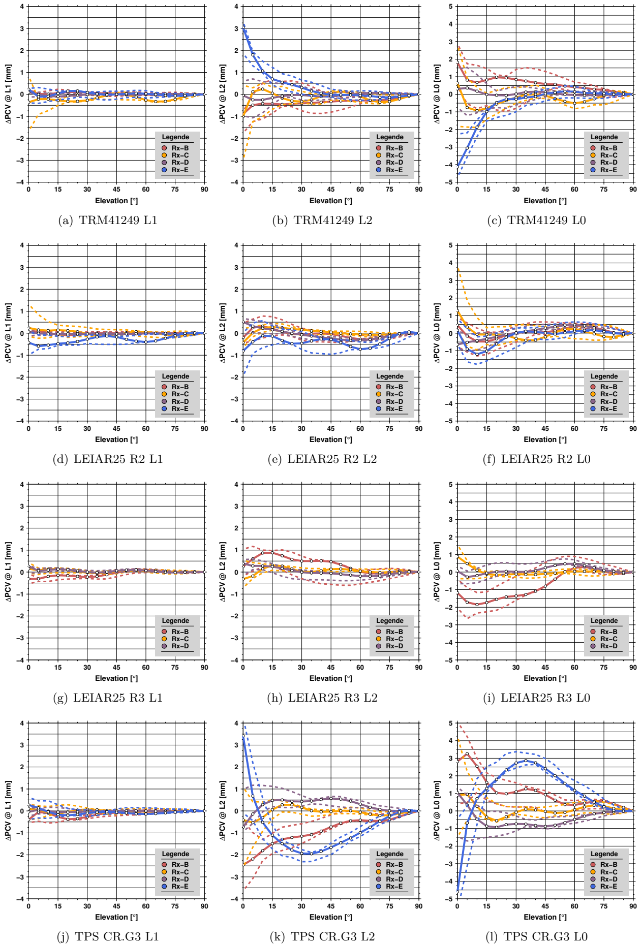
Abbildung 6.20: Einfluss verschiedener Referenzstationsempfänger auf die GPS PCV Schätzung. Die getrichelten Linien zeigen das Maximum und Minimum der Variationen im Azimut.
