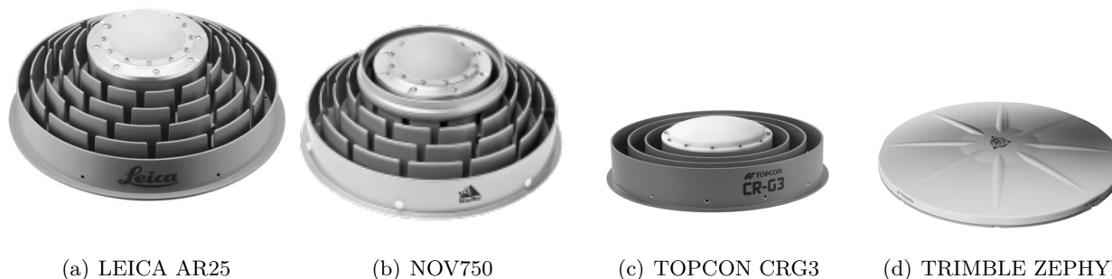
Abbildung 6.19: Im Rahmen der Versuchsreihe verwendete GNSS-Antennen. Abbildung (b) zeigt eine Novatel NOV750, die jedoch baugleich zur Leica AR25.R3 ist.
