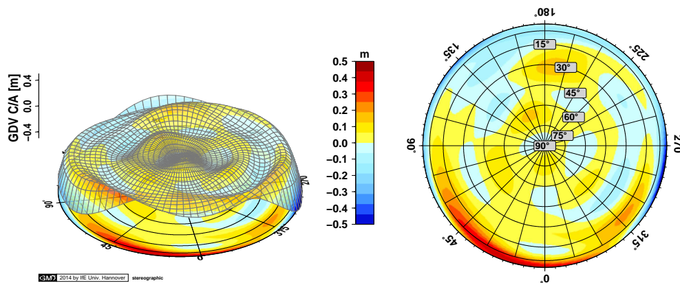
(b) Differenz der aufeinander korrigierten GPS C/A GDV bei siderischer Wiederholung
