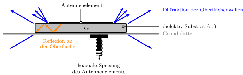
Abbildung 2.13: Oberflächenwellen sowie Reflexions- und Diffraktionsphänomene an Mikrostreifenantennen.
