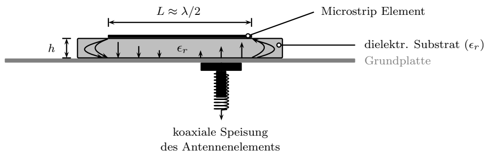
Abbildung 2.7: Erzeugung der Polarisation zwischen Substrat und Mikrostrip Element (Antennenelement); die Speisung der Antenne erfolgt durch die Grundplatte.
