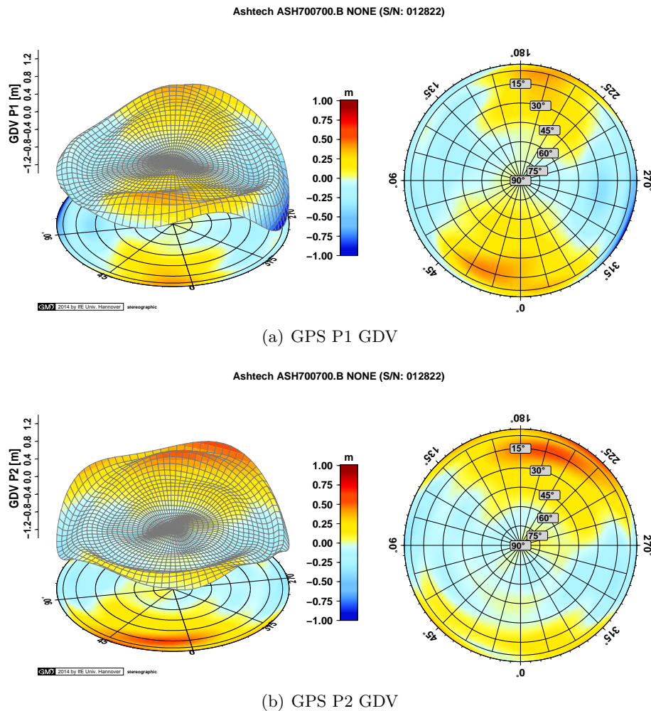
Abbildung 5.3: Ergebnisse der GDV Antennenkalibrierung auf den Codephasen P1 und P2 für eine Ashtech Marine Antenne ASH700700.B NONE für GPS P1 (a) GPS P2 (b).
