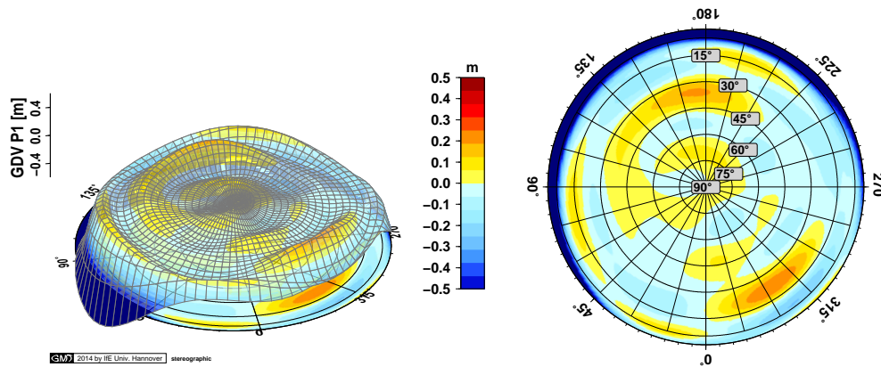
(c) Differenz der aufeinander korrigierten GPS P1 GDV bei siderischer Wiederholung
