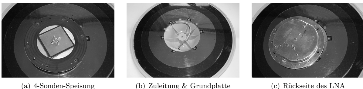
Abbildung 2.10: Speisungstechnik (4-Probe) bei einer Trimble Zephyr I Geodetic, (geöffnet 2008 durch IfE).
