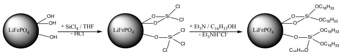
Abb. 8-1: Organofunktionalisierung von \text{LiFePO}_4 mittels \text{SiCl}_4 und 1-Hexadecanol unter Verwendung von Triethylamin als Base (schematisch).
