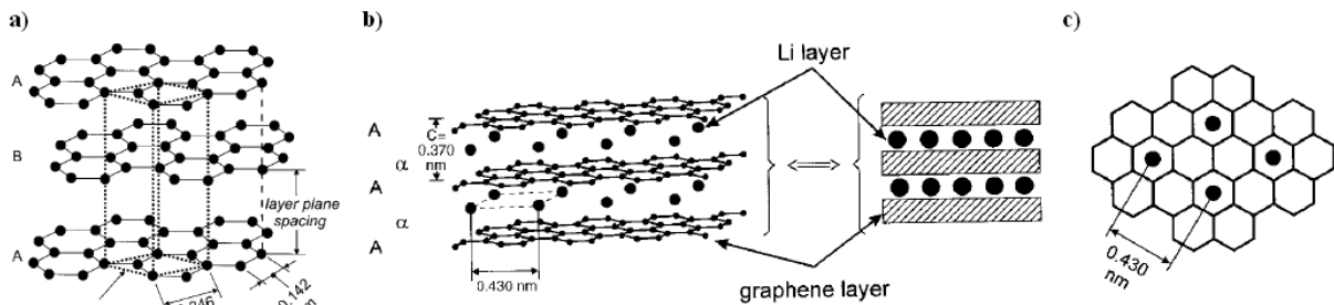
Abb. 2-3: Schichtstrukturen des Graphits (a) ABA-Schichtfolge, (b) AAA-Schichtfolge und (c) Querschnitt der LiC 6 -Einheiten. [2]
