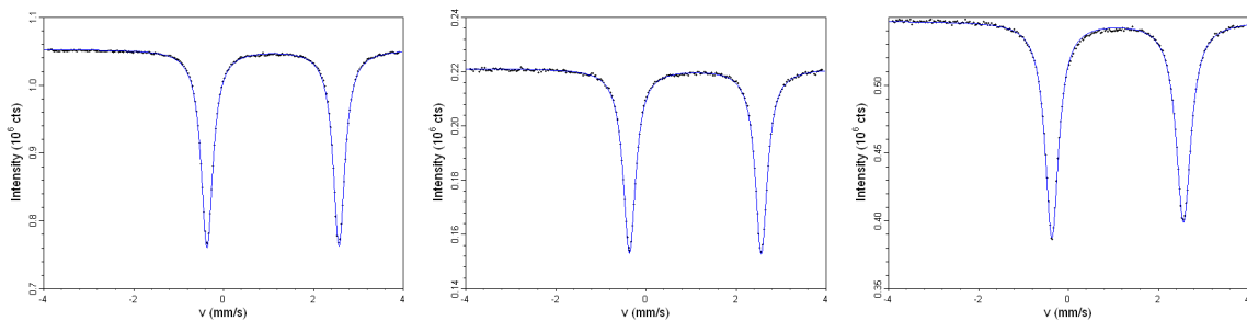
Abb. 9-2: Experimentell erhaltene Messdaten (schwarz), simulierte Signale (blau) der \text{LFP}_{\text{FK}} (o/p 1 ) (links), \text{LFP}_{\text{FK}} (o/p 2 ) (Mitte) und \text{LFP}_{\text{FK}} (o/p 3 ) (rechts).
