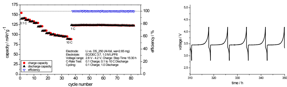
Abb. 9-17: C-Ratentest des LFP FK (o/p 3 ) (links) und Zyklovoltogramm (rechts).
