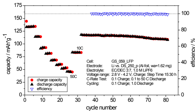
Abb. 9-18: C-Ratentest des LFP FK (o/p 3 ) mit einer gepressten Elektrode.
