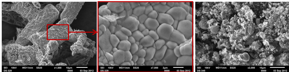
Abb. 7-22: REM-Aufnahmen der synthetisierten Produkte aus Eisencitrat und \text{LiH}_2\text{PO}_4 mit einer Reaktionszeit von 3 h und einer Reaktionstemperatur von 800 °C (links und Mitte) und 900 °C (rechts).
