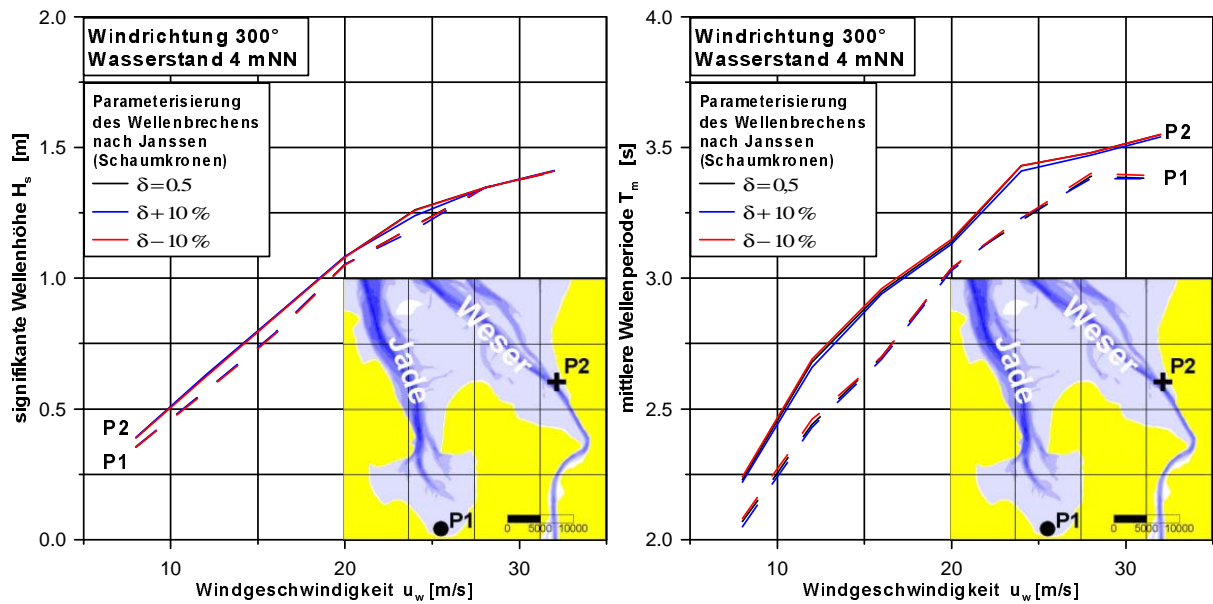
Abbildung I-5: Seegangbedingungen vor der Küste nahe Jade-Wapeler-Siel (P1) und nahe Wremertief (P2) für einen Sturmflutwasserstand von NN + 4 mNN und Wind aus nordwestlichen Richtungen bei einer Unsicherheit in dem das steilheitsinduzierte Wellenbrechen beschreibenden Parameter \delta von \pm 10\% um den Standardwert von 0,5 – signifikante Wellenhöhe (links) und mittlere Wellenperiode (rechts) –
