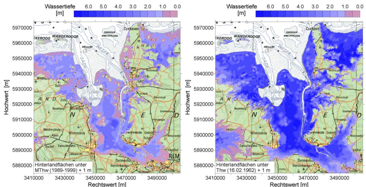
Abbildung 5-2: Bei Wasserstandsanstieg um 1 m unter MThw (links) bzw. dem um 1 m erhöhten Thw der Sturmflut vom 16.02.1962 liegende Flächen im Jade-Weser-Gebiet (Datengrundlage: DGM 50)
