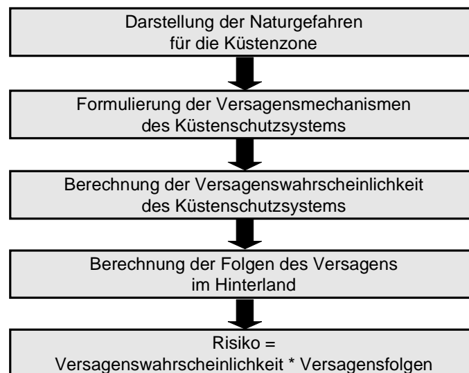
Abbildung 3-3: Arbeitsschritte einer Risikoanalyse für die Küstenzone [ZIMMERMANN UND MAI, 1998, nach VERGEER, 1990]
