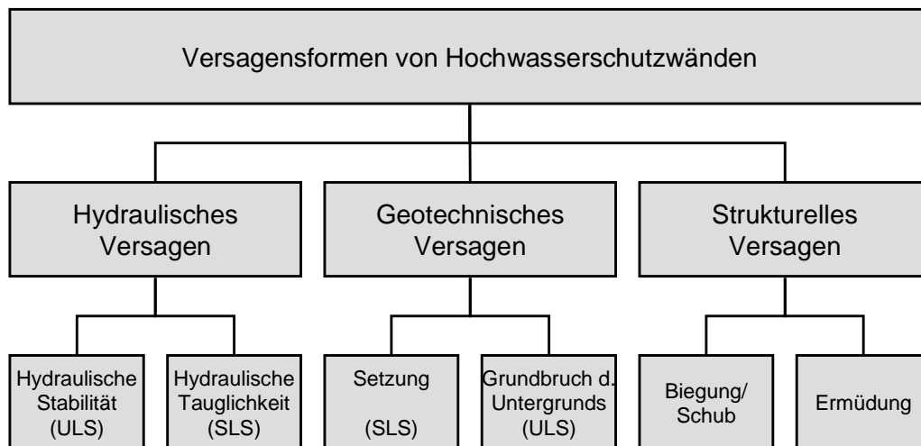
Abbildung 3-18: Hauptversagensmechanismen von Hochwasserschutzwänden [vgl. OUMERACI ET AL., 2001].
