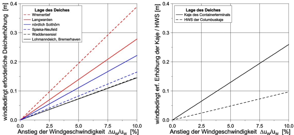
Abbildung 4-63: Erforderliche Erhöhung verschiedener Deiche am Jade-Weser-Ästuar (links) sowie der Kaje des Containerterminals bzw. der Hochwasserschutzwand der Columbuskaje in Bremerhaven (rechts) zur Aufrechterhaltung des derzeitigen Sicherheitsniveaus in Abhängigkeit von der Intensivierung des Windes
