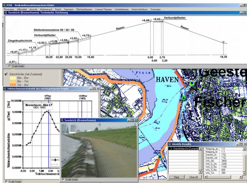
Abbildung R-5: RISK – Kataster der Hauptdeiche
