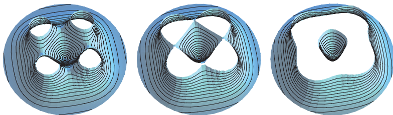
Abbildung 2.6.: Effektives Potential für die xy -Ebene eines linearen Quadrupols mit zylindrischen Stabradien mit (von links nach rechts) r_s/r_0 \approx 0.6, 1.1, 1.4
