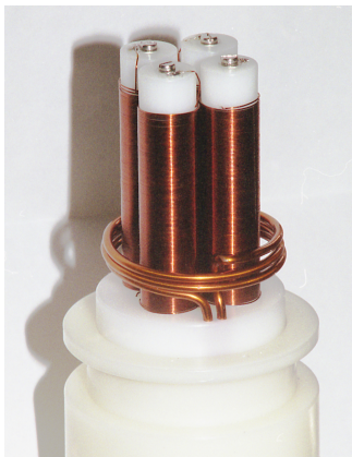
Abbildung 3.26.: Kernloser Resonanztransformator
