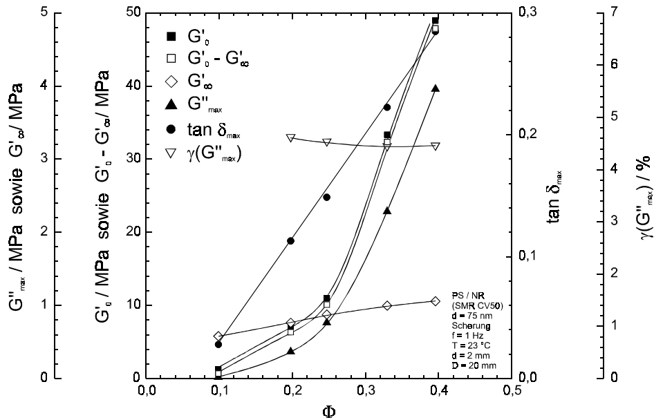
Abb. 29: Dynamische Eigenschaften (Schерung) PS-Mikrogel-gefüllter NR-Vulkanisate in Abhängigkeit vom Füllstoffvolumenbruch.
