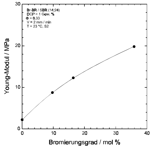
Abb. 155: Zugversuch an Br-BR-Mikrogel-gefüllten SBR-Vulkanisaten ( \Phi = 0,33 ), Variation des Bromierungsgrads [mol %] der Mikrogele.
