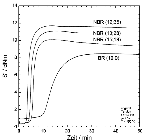
Abb. 4: Vulkanisationsisothermen in Abhängigkeit des Kautschuknitrilgehalts.
