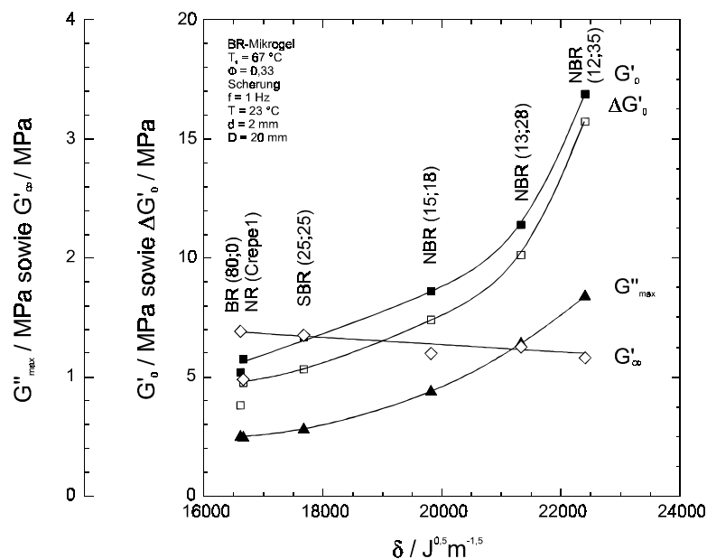
Abb. 75: Dynamische Eigenschaften (Scherung) BR-Mikrogel-gefüllter Vulkanisate in Abhängigkeit des Kautschuk- \delta -Parameters ( T_g = 67 \text{ }^\circ\text{C} , \Phi = 0,33 ).
