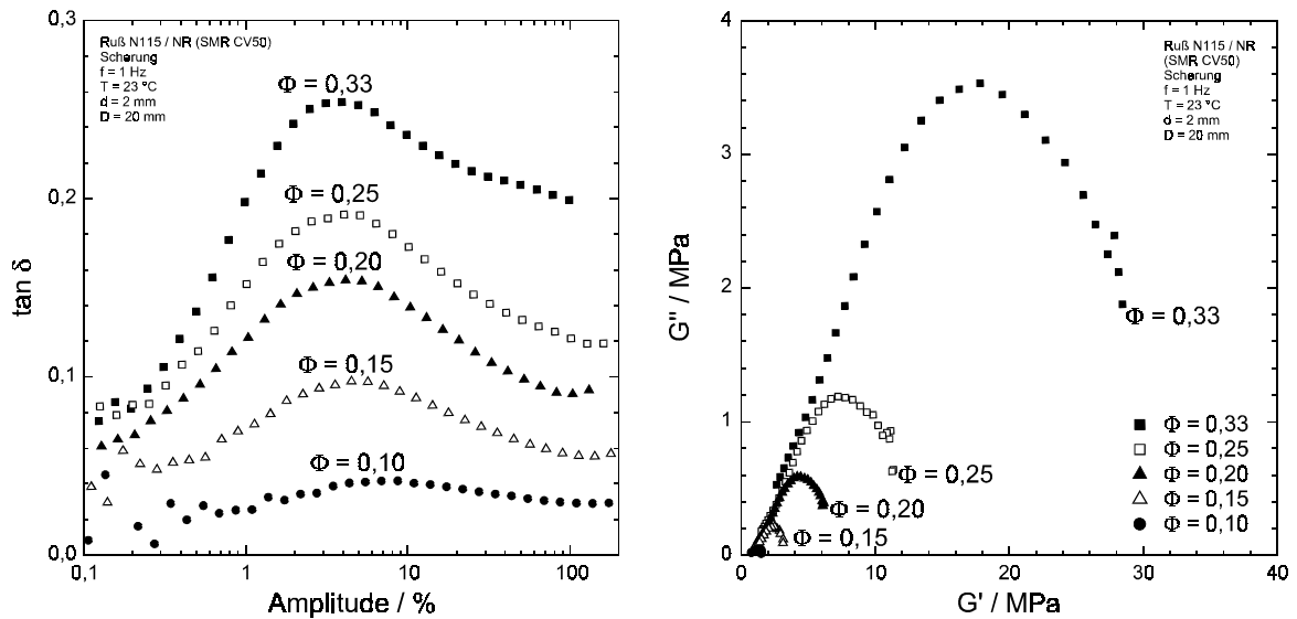
Abb. 22: Verlustfaktor (Scherung) Ruß N115-gefüllter NR-Vulkanisate in Abhängigkeit der Deformation, Variation des Füllstoffvolumenbruchs.
