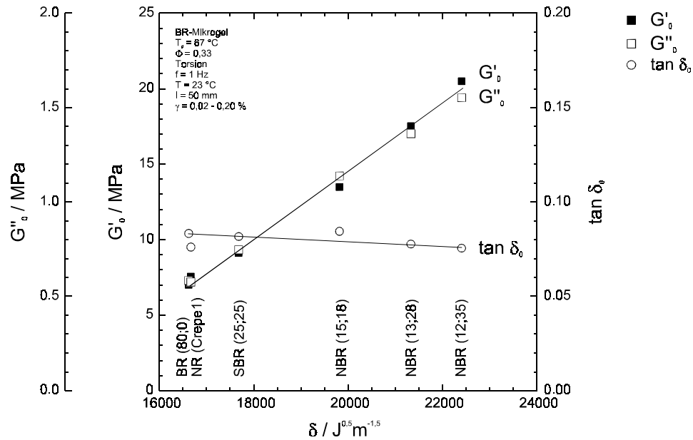
Abb. 70: Dynamische Eigenschaften (Torsion) von BR-Mikrogel-gefüllten Vulkanisaten in Abhängigkeit des Kautschuk- \delta -Parameters ( T_g = 67 \text{ }^\circ\text{C} , \Phi = 0,33 ).
