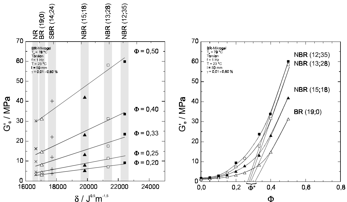
Abb. 66: Dynamischer Speichermodul (Torsion) von BR-Mikrogel-gefüllten Vulkanisaten in Abhängigkeit des Kautschuk \delta -Parameters (BR: T_g = 79^\circ\text{C} ).
