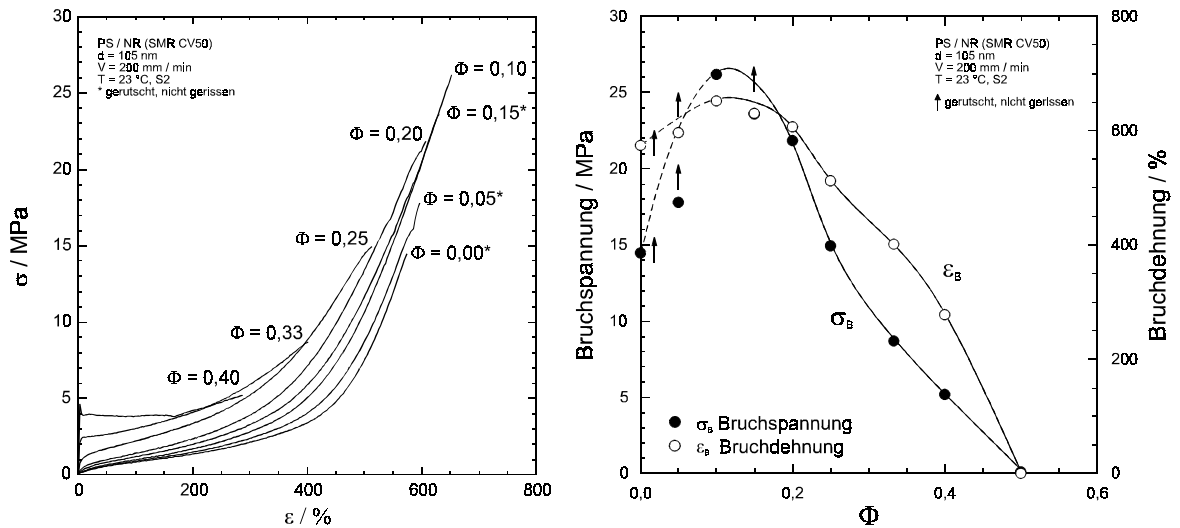
Abb. 35: Zugversuch an PS-Mikrogel-gefüllten NR-Vulkanisaten, Variation des Füllstoffvolumenbruchs.
