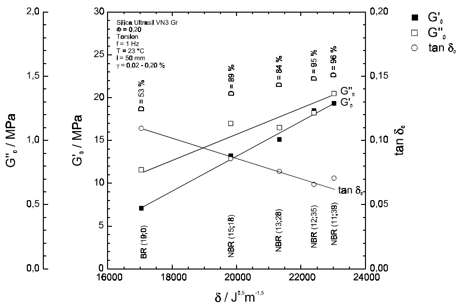
Abb. 88: Dynamische Eigenschaften (Torsion) von Kieselsäure Ultrasil VN3 Gr-gefüllten Vulkanisaten in Abhängigkeit des Kautschuk- \delta -Parameters.
