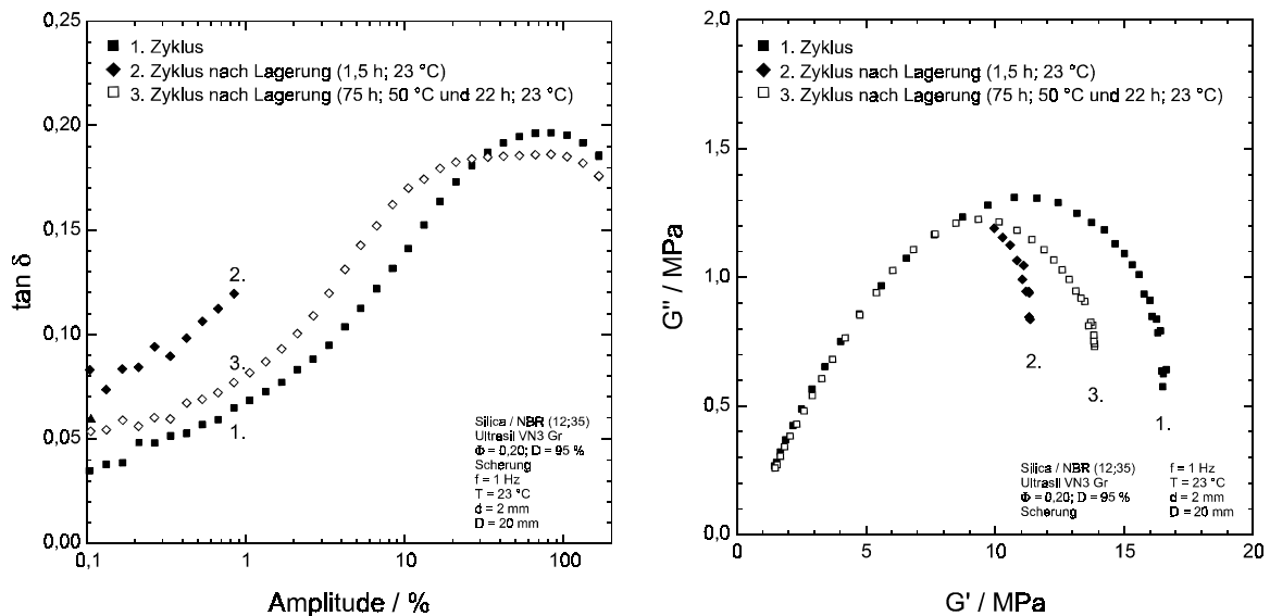
Abb. 10: Verlustfaktor (Scherung) Kieselsäure-gefüllter NBR-Vulkanisate in Abhängigkeit der Deformation und der Rückerholung ( \Phi = 0,20 ).
