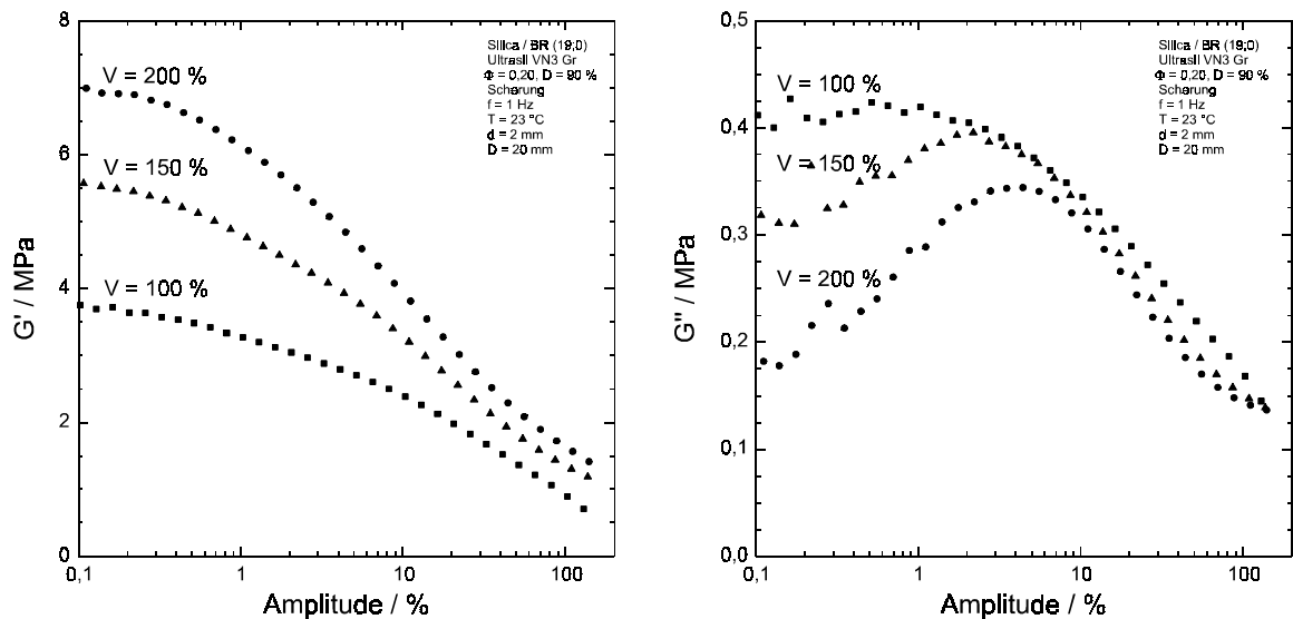
Abb. 57: Dynamischer Speichermodul (Schерung) Kieselsäure-gefüllter BR-Vulkanisate in Abhängigkeit der Deformation, Variation der Vernetzerdosierung [V / %].
