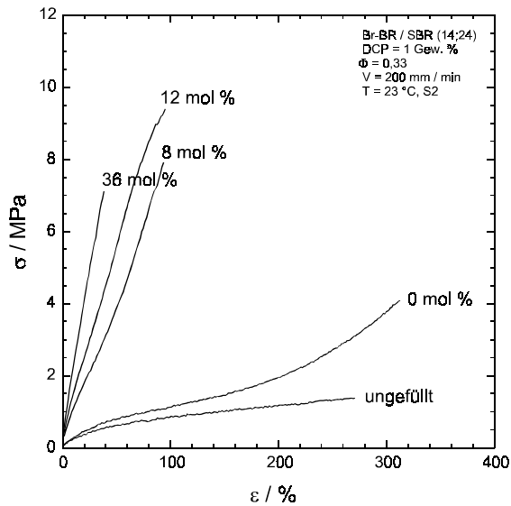
Abb. 155: Zugversuch an Br-BR-Mikrogel-gefüllten SBR-Vulkanisaten ( \Phi = 0,33 ), Variation des Bromierungsgrads [mol %] der Mikrogele.
