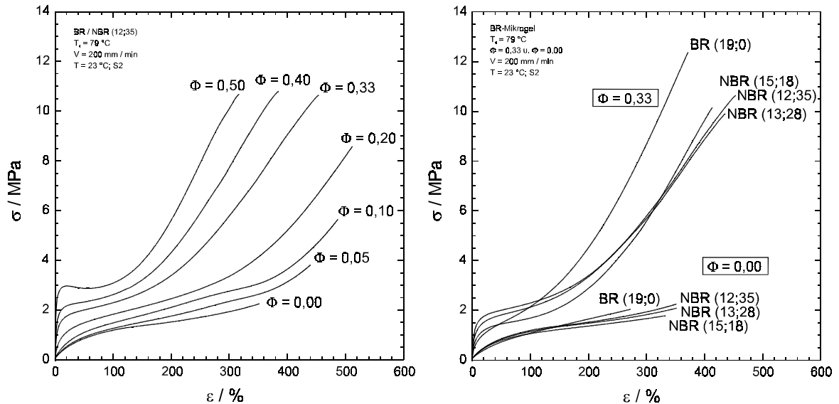
Abb. 76: Zugversuch, Volumenbruchvariation BR-Mikrogel-gefüllter NBR-Vulkanisate [BR: T_g = 79^\circ\text{C} , NBR (12;35)].
