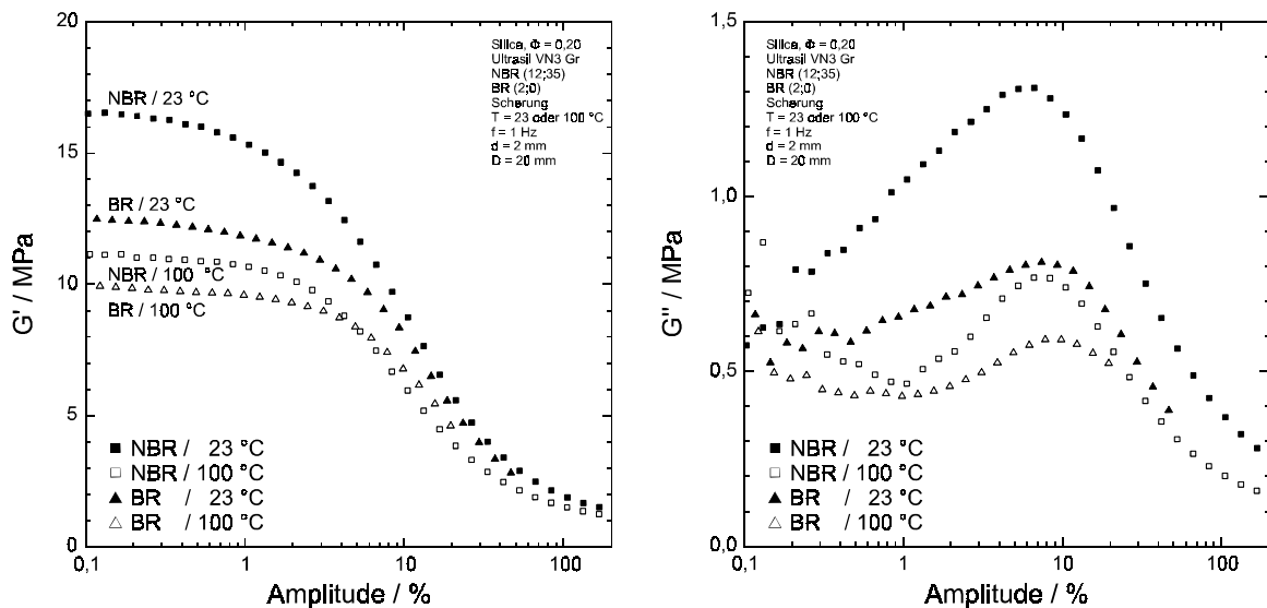
Abb. 99: Dynamischer Speichermodul (Scherung) Kieselsäure-gefüllter Vulkanisate in Abhängigkeit der Deformation, Kautschuk- u. Temperaturvariation ( \Phi = 0,20 ; Ultrasil VN3 Gr).
