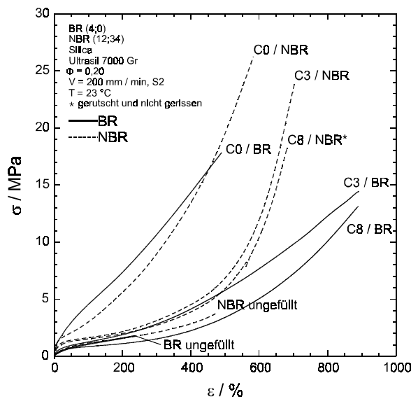
Abb. 147: Zugversuch an Kieselensäure-gefüllten NR-Vulkanisaten, Variation der Kieselensäuremodifizierung ( \Phi = 0,20 ).
