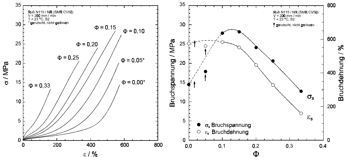
Abb. 32: Zugversuch an Ruß N115-gefüllten NR-Vulkanisaten, Variation des Füllstoffvolumenbruchs.
