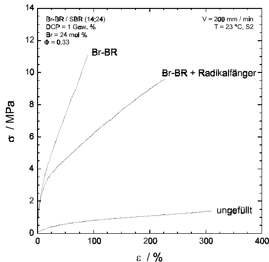
Abb. 165: Zugversuch an Br-BR-Mikrogele gefüllten SBR-Vulkanisaten ( \Phi = 0,33 ) in Gegenwart und Abwesenheit von Radikalfängern.
