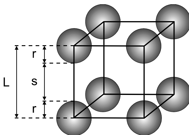
Abb. 113: Elementarzelle des kubisch primitiven Gitters.
