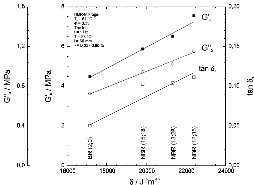
Abb. 78: Dynamische Eigenschaften (Torsion) von NBR-Mikrogel-gefüllten Vulkanisaten in Abhängigkeit des Kautschuk- \delta -Parameters ( T_g = 61 \text{ }^\circ\text{C} , \Phi = 0,33 ).
