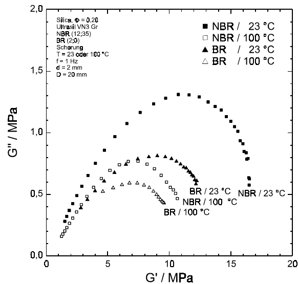
Abb. 101: COLE-COLE-Darstellung der dynamischen Moduli (Schерung) Kieselsäuregefüllter Vulkanisate in Abhängigkeit des Kautschuks (NBR (12;35), BR (2;0)) und der Temperatur (Ultrasil VN3 Gr).
