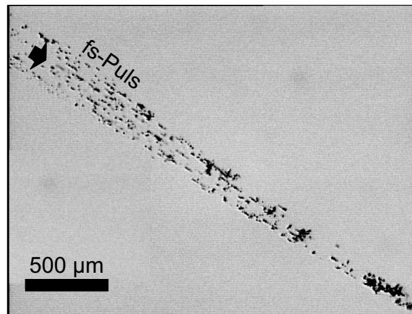
Abbildung 5.5.: Filamentierung in PMMA. Die einzelnen Durchbruchstellen sind innerhalb einzelner Filamente sichtbar.
