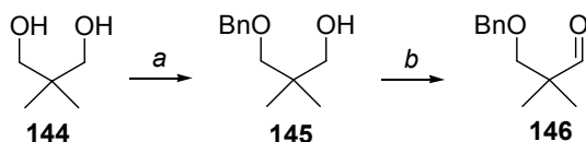
Abb. 67 Synthese des Aldehyds 146 : (a) BnCl, t -BuOK, Dioxan, Rückfluss, 80%; (b) SO 3 ·Py, DMSO, Et 3 N, DCM, 0 °C, 86%.
