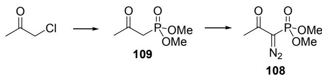
Abb. 53 Herstellung des Ohira Bestmann Reagenzes
