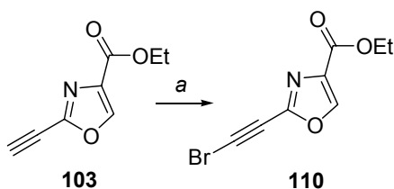
Abb. 54 Synthese des Bromalkins 110 : (a) NBS, AgNO 3 , Aceton, RT, 84%.
