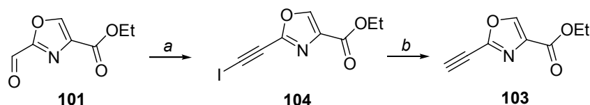
Abb. 51 Generierung von Oxazolalkin 103 über Iodalkin 104 (a) \text{CHI}_3 , t -BuOK, DCM, RT, 80%; (b) n -BuLi, -100\text{ }^\circ\text{C} , \text{NH}_4\text{Cl} , 40%.
