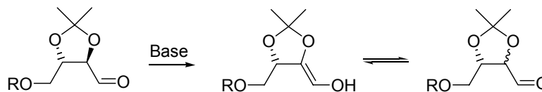
Abb. 63 Baseninduzierte teilweise Racemisierung nach Sharpless et al.
