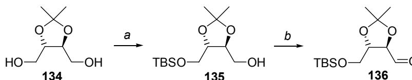
Abb. 62 Darstellung von Aldehyd 136 : (a) NaH, TBSCl, THF, RT, 85%; (b) \text{SO}_3\cdot\text{Py} , DMSO, \text{Et}_3\text{N} , DCM, 0\text{ }^{\circ}\text{C} , 96%.
