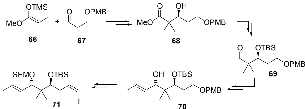
Abb. 31 Synthese des C11-C19 Fragments von Disorazol C 1 nach I. V. Hartung
