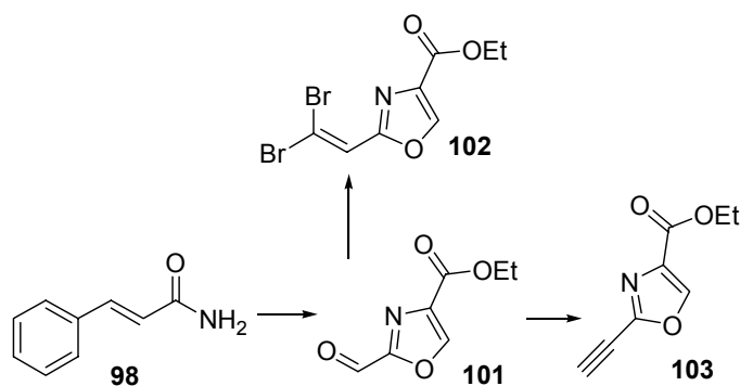
Abb. 86 Synthese des Oxazolalkins 103
