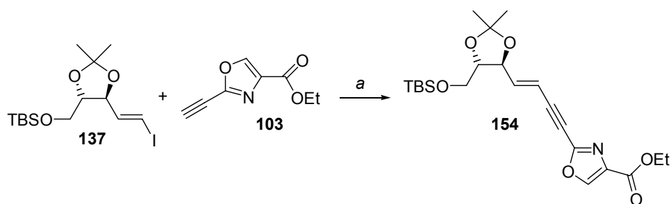
Abb. 74 Synthese des C1-C11 Fragments 154 von Disorazol D 1 : (a) Pd(PPh 3 ) 2 Cl 2 , CuI, DMF, dann 137 , Et 3 N, 45 min, RT, dann 103 in DMF, 86 %.
