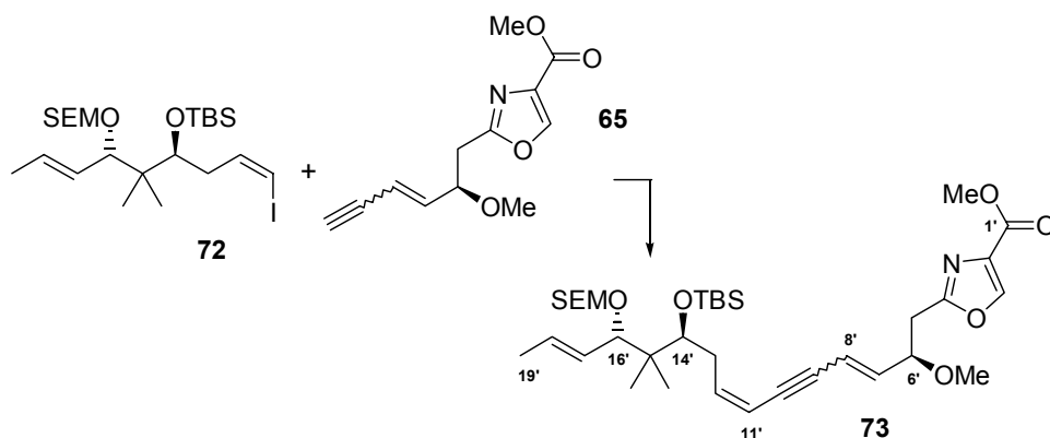
Abb. 32 Synthese der maskierten Disorazol C 1 Hälfte
