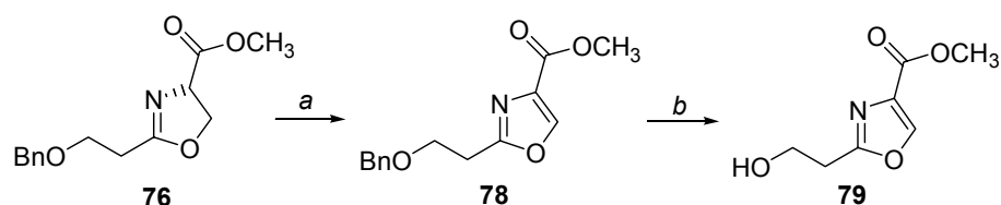
Abb. 35 Darstellung des Alkohols 79 : (a) DBU, Py, CCl 4 , CH 3 CN, RT, 68%; (b) H 2 , Pd/C, EtOH, RT, 12 h, 86%.
