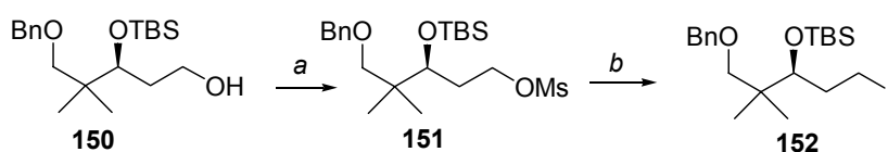
Abb. 70 Synthese des Iodids 152 : (a) MsCl, DMAP, Et 3 N, THF, 0 °C, 93% ; (b) NaI, Acetone, NaHCO 3 , Rückfluss, 3 h, 78%.
