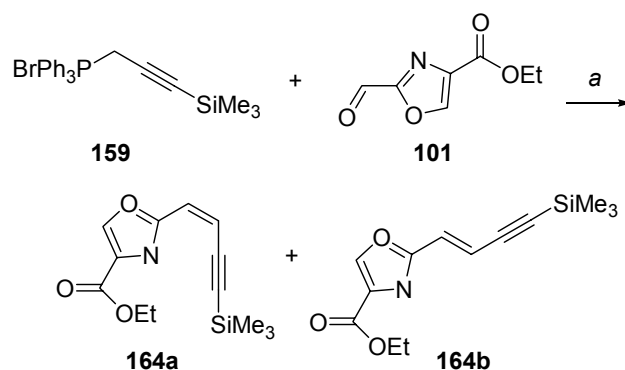
Abb. 81 Disorazol Derivatisierungen – C_2 -Verlängerung: (a) n -BuLi, THF, -78 °C, 1.5 h, 16 %, E/Z, 1/1.5.
