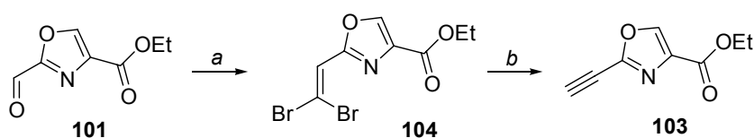
Abb. 50 Corey-Fuchs-Homologisierung zum Oxazolalkin 103 : (a) CBr 4 , PPh 3 , DCM, RT, 70%; (b) n-BuLi, THF, -78 °C, 30%.
