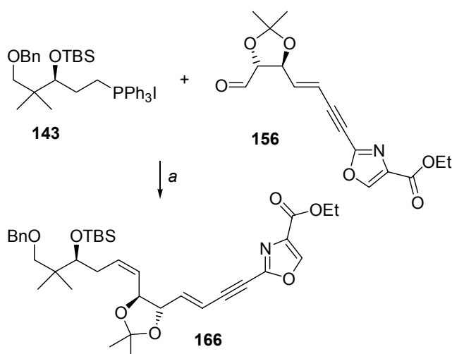
Abb. 83 Generierung eines Modells für die Macrocyclisierung: (a) NaHMDS, THF, -78\text{ }^{\circ}\text{C} , 4h, 28%, Z/E, 5/1.
