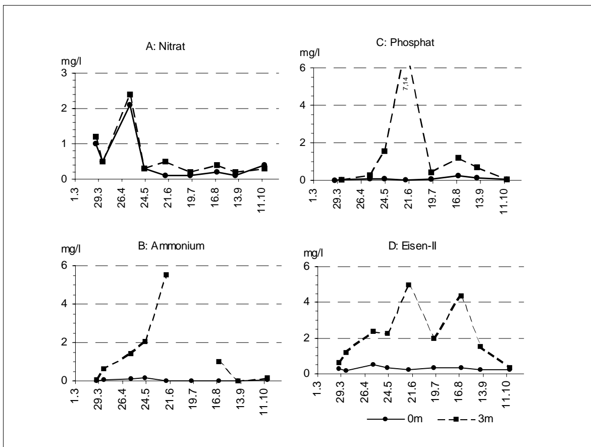
Abb. 29: Konzentrationsverlauf der Trophieparameter Nitrat (A), Ammonium (B), Phosphat (C) sowie Eisen (D) im Kleinen Heiligen Meer während der Vegetationsperiode 1998. Jeweils zum 6. Mai, 17. Juni und 18. August 1998 fand eine Durchmischung der Wassermassen statt.
