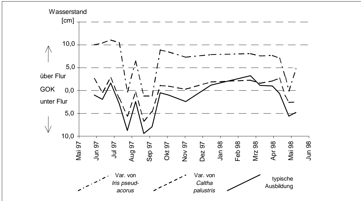
Abb. 24: Wasserstandsganglinien im Erlenbruchwald am Südost- und Ostufer des Großen Heiligen Meeres (erweitert nach ROLFES 1998).
