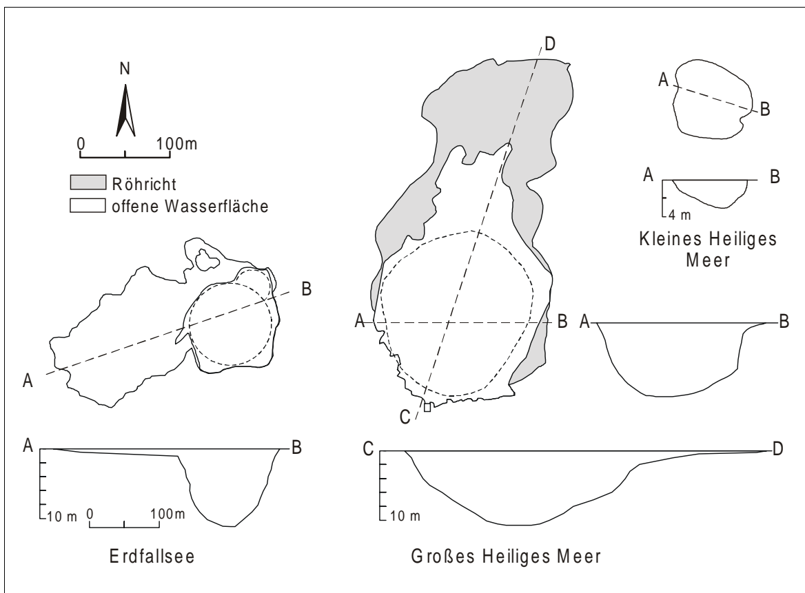
Abb. 2: Morphologie der Gewässer Erdfallsee und Großes Heiliges Meer (nach LOTZE 1957, verändert) sowie des Kleinen Heiligen Meeres (eigene Lotung) im maßstabgetreuen Vergleich. Die unterbrochenen Linien deuten die Erdfalltrichter an, die punktierten Linien stellen die Schnittebenen der Tiefenprofile dar. Diese sind 10fach überhöht.
