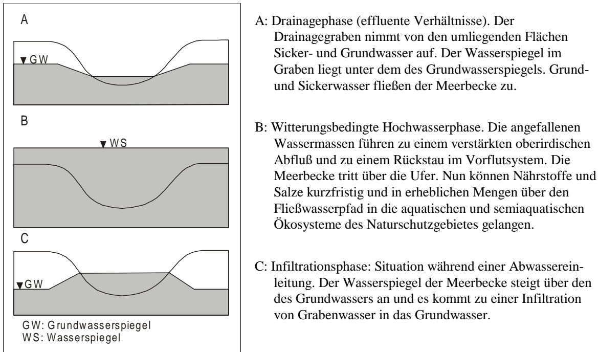
Abb. 33: Schematische Darstellung der Wasserführung und der Vorflutsituation in der Meerbecke. Beziehung der Stände vom Grundwasser (GW) und des Wassers der Meerbecke (WS) in Abhängigkeit von der jeweiligen Wasserführung (nach HAGEMANN & PUST 1999).
