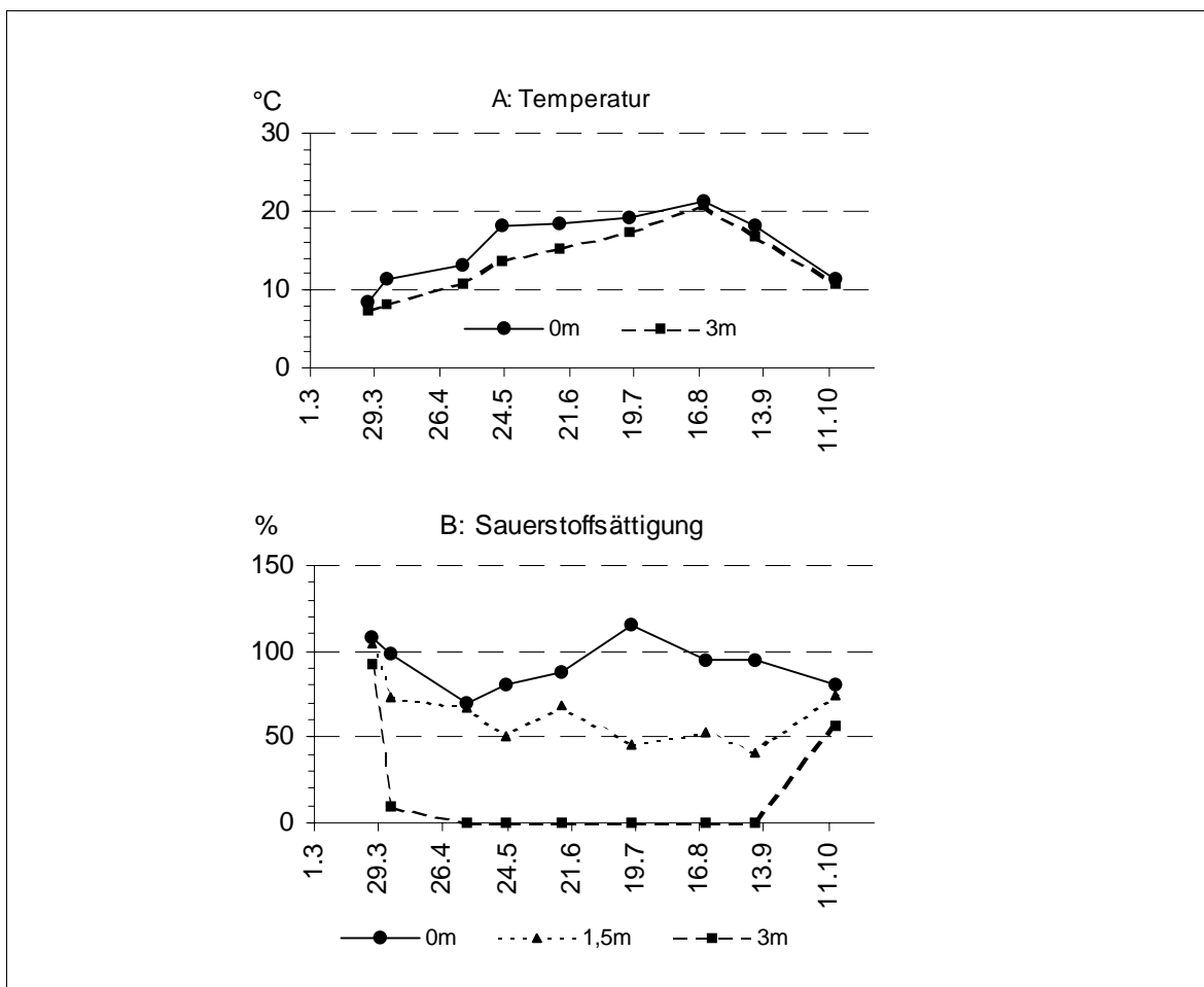
Abb. 28: Veränderungen der Temperatur (A) und der Sauerstoffsättigung (B) im Kleinen Heiligen Meer während der Vegetationsperiode 1998. Jeweils zum 6. Mai, 17. Juni und 18. August 1998 fand eine Durchmischung der Wassermassen statt.
