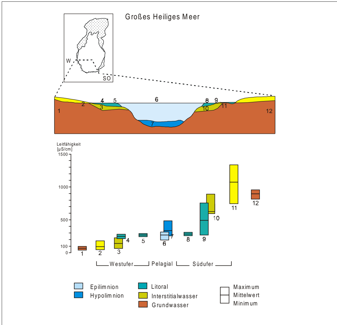
Abb. 27: Schematischer Schnitt durch das Große Heilige Meer. Dargestellt ist eine Differenzierung verschiedener Uferabschnitte mit Hilfe der Leitfähigkeit als Summenparameter für die Trophie, (1- Grundwasser (GWM 22); 2- Bodenwasser (W3); 3- Interstitialwasser am Westufer (WI); 4- Freiwasser am Westufer (W1); 5- Freiwasser in der Schwimmblattzone am Westufer (GW); 6- Freiwasser Pelagial (Mittelwert 0-3m); 7- Freiwasser Pelagial (Mittelwert 8-10m); 8- Freiwasser in der Schwimmblattzone am Südufer (GS1); 9- Freiwasser am Südufer (S1); 10- Interstitialwasser am Südufer (SI); 11- Bodenwasser am Südufer (S4); 12- Grundwasser (GWM 6)).
