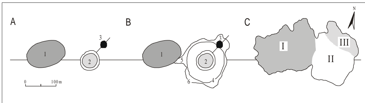
Abb. 1: Genese des Erdfallsees (nach TIETZE 1914 und SCHROEDER 1957, verändert aus HÖLTER 1998)
