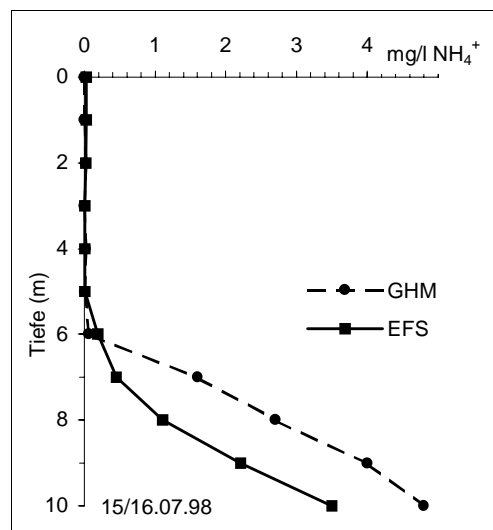
Abb. 11: Ammoniumkonzentration im Tiefenprofil vom 15/16.7.98 als Beispiel für eine unterschiedlich intensive Nährstoffrücklösung aus dem Sedimenten des Erdfallsees und des Großen Heiligen Meeres.
