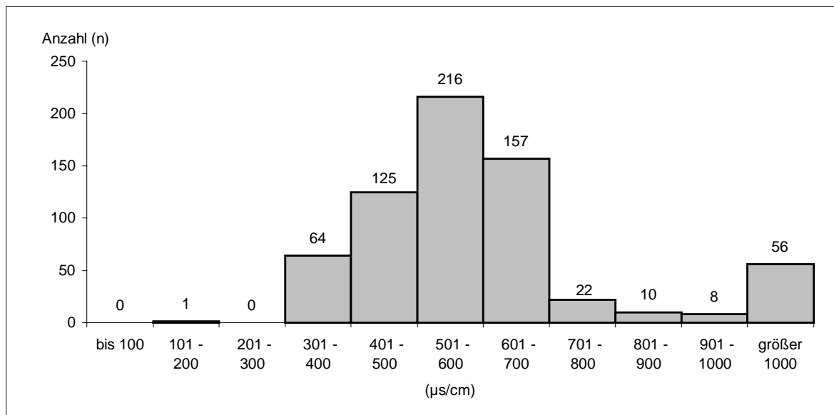
Abb. 32: Häufigkeitsverteilung (auf der Basis von täglichen Messungen) der Leitfähigkeit ( \mu\text{S}/\text{cm} ) in der Meerbecke für den Zeitraum Oktober 1996 bis Dezember 1998.
