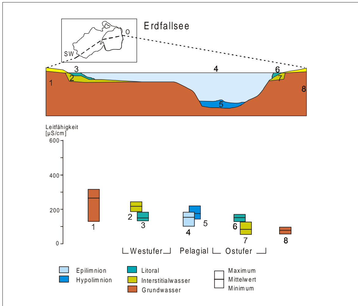
Abb. 25: Schematischer Schnitt durch den Erdfallsee. Dargestellt ist eine Differenzierung verschiedener Uferabschnitte mit Hilfe der Leitfähigkeit als Summenparameter für die Trophie, (1- Grundwasser (GWM 16); 2- Interstitialwasser am Westufer (EW1A); 3- Freiwasser am Westufer (EW1); 4- Freiwasser Pelagial (Mittelwert 0-3m); 5- Freiwasser Pelagial (Mittelwert 8-10m); 6- Freiwasser am Ostufer (EO); 7- Interstitialwasser am Ostufer (EO2); 8- GWM 23).
