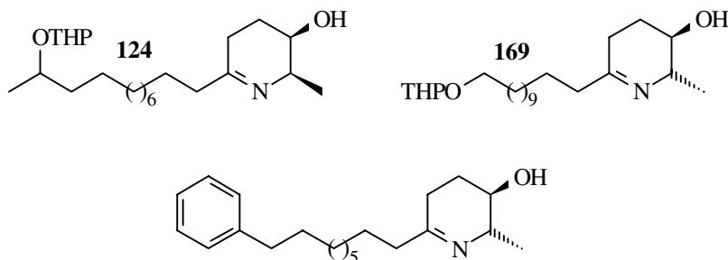
Abb. 4.8: Iminvorläufer
