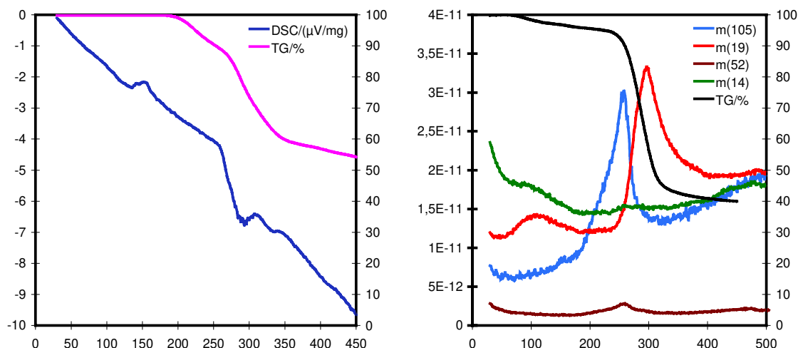
Abb. 29: Thermisches Verhalten des Komplexes \text{Eu}[(\text{CH}_3\text{NHO})\text{C}_6\text{H}_5\text{COCH}_2\text{COCF}_3]_3 \cdot 2\text{H}_2\text{O} , linke Abbildung: DSC/T und TG/T-Diagramme rechte Abbildung: TG/T-Diagramm im Vergleich mit der MS-Messung
