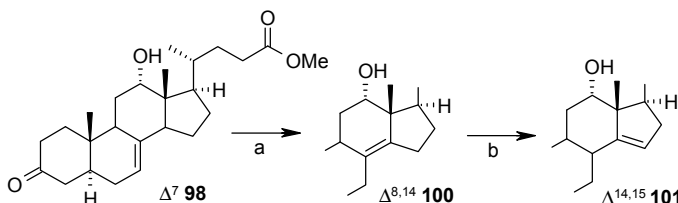
Schema 54: Umlagerung des \Delta^7 -5 \alpha -Cholans 98
