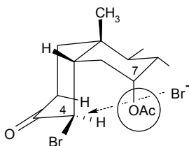
Abb. 8: Behinderung der Bromid-Einflugschneise durch das 7 \alpha -Acetat
