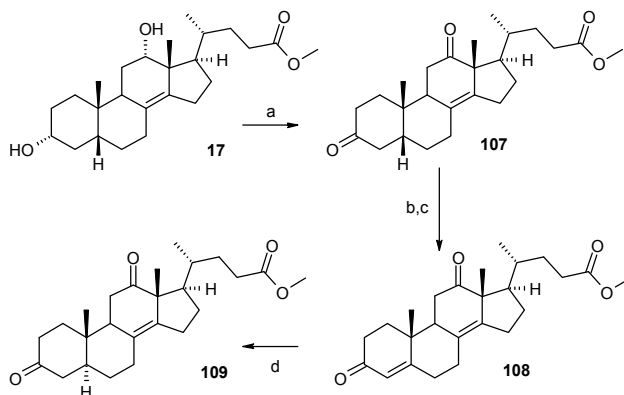
Schema 56: Synthese des \Delta^{8,14} -5 \alpha -Diketons 109
