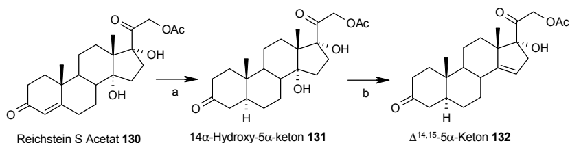
Schema 72: Synthese des \Delta^{14,15} - 5\alpha -Ketons 132
