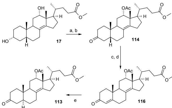
Schema 59: Synthese von \Delta^{8,14} -5 \alpha -12-Acetat 113
