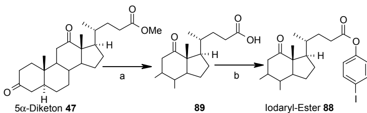
Schema 48: Darstellung des Iodaryl-Esters 88
