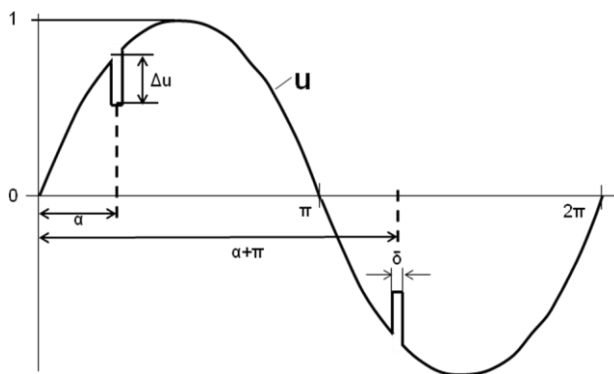
Bild 3: Kommutierungseinbrüche in der Spannung
