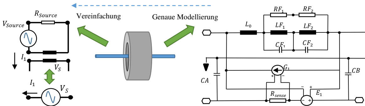
Abbildung 3: Vereinfachung - BCI-Modell
