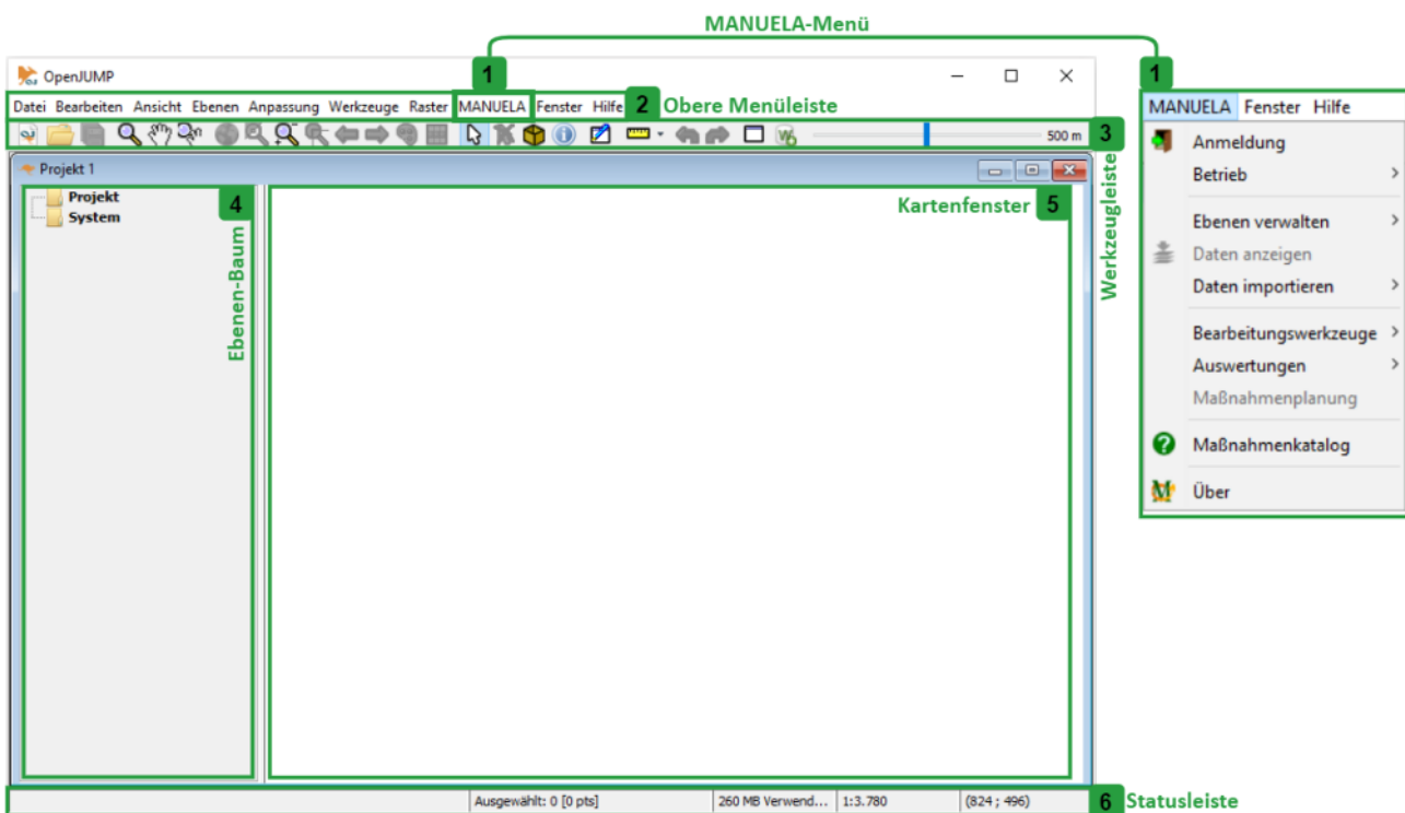
Abbildung 5: Übersicht der OpenJUMP-Benutzeroberfläche
