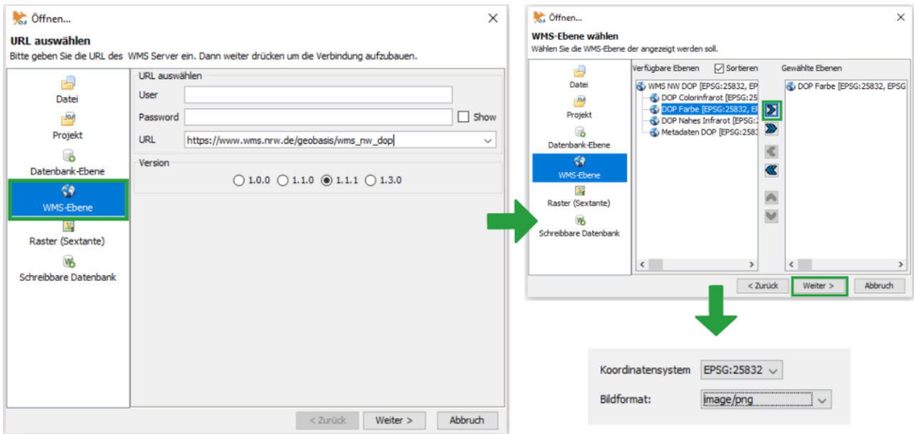
Abbildung 16: WebMapService in OpenJUMP einbinden
