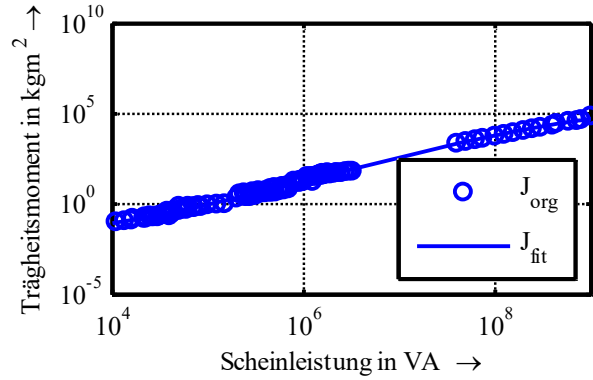
Abbildung 32: Massenträgheitsmoment in Abhängigkeit von der Bemessungsscheinleistung (Punkte: originale Beispieldaten; Linie: angenäherte Annahme)
