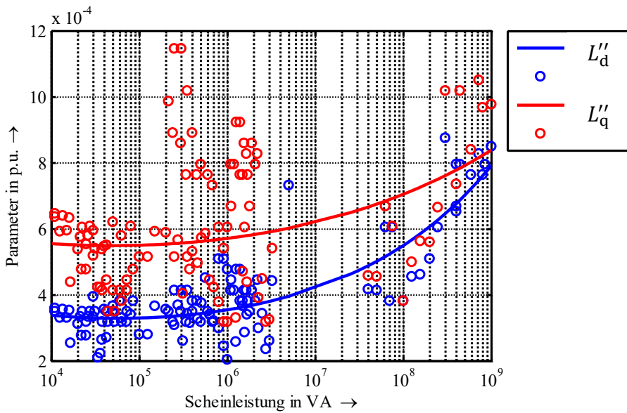
Abbildung 33: Subtransiente Induktivitäten der d- und q-Achse in Abhängigkeit von der Bemessungsscheinleistung (Punkte: originale Beispieldaten; Linie: angenäherte Annahme)
