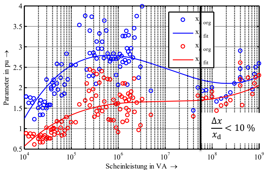
Abbildung 102: Stationäre Reaktanzen der d- und q-Achse in Abhängigkeit von der Bemessungscheinleistung (Punkte: originale Beispieldaten; Linie: approximierte Annahme)
