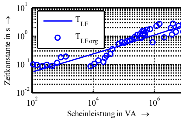
Abbildung 42: Läuferzeitkonstante in Abhängigkeit von der Bemessungsscheinleistung (Punkte: originale Beispieldaten; Linie: approximierte Annahme)
