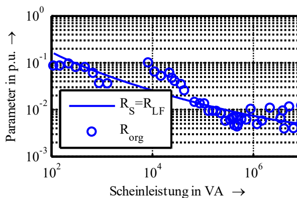
Abbildung 39: Ständerwiderstand in Abhängigkeit von der Bemessungsscheinleistung (Punkte: originale Beispieldaten; Linie: approximierte Annahme)
