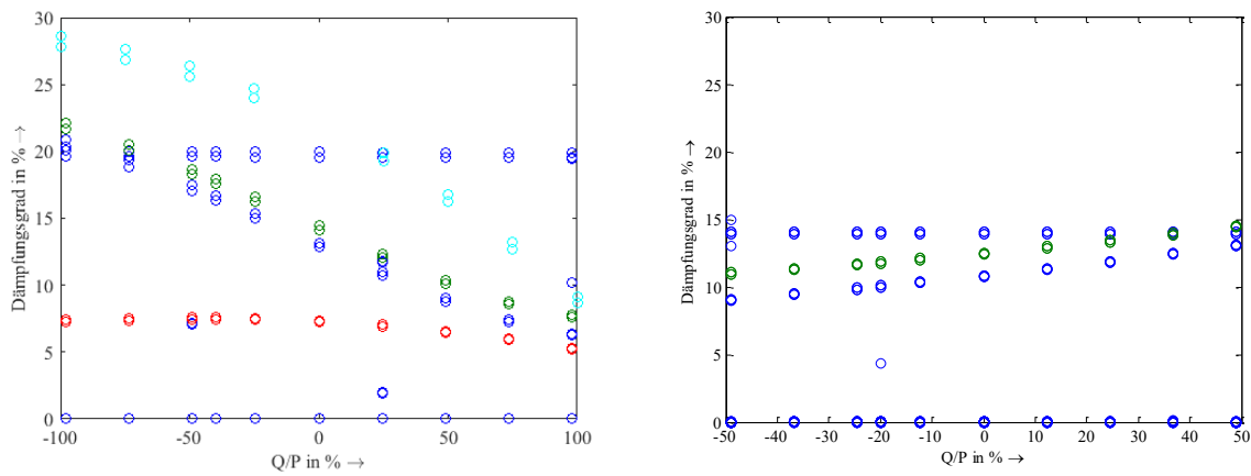
Abbildung 95: Abhängigkeit des Dämpfungsgrades von der Blindleistungsbereitstellung bei Synchronmaschinen (links: blau=sub-RL, grün=sub-RLq, türkis=tra-RLq, rot=tram-RLq) und bei Asynchronmaschinen (rechts: blau=tra.RL, grün=tra-RLq) im Mittelspannungsnetz (MS)
