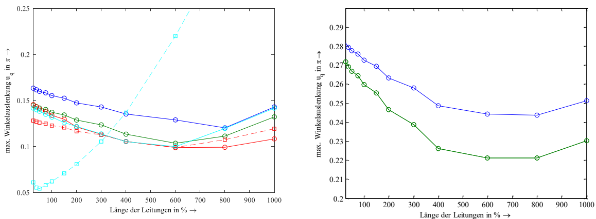
Abbildung 84: Abhängigkeit des maximalen Spannungswinkels von der Leitungslänge bei Synchronmaschinen (links: blau=sub-RL, grün=sub-RLq, türkis=tra-RLq, rot=tram-RLq) und bei Asynchrongeneratoren (rechts: blau=tra.RL, grün=tra-RLq) im Mittelspannungsnetz (MS)
