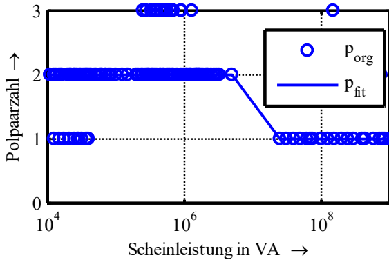
Abbildung 31: Polpaarzahl in Abhängigkeit von der Bemessungsscheinleistung (Punkte: originale Beispieldaten; Linie: angenäherte Annahme)
