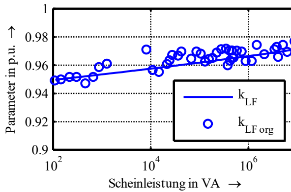
Abbildung 41: Koppelfaktor in Abhängigkeit von der Bemessungsscheinleistung (Punkte: originale Beispieldaten; Linie: approximierte Annahme)
