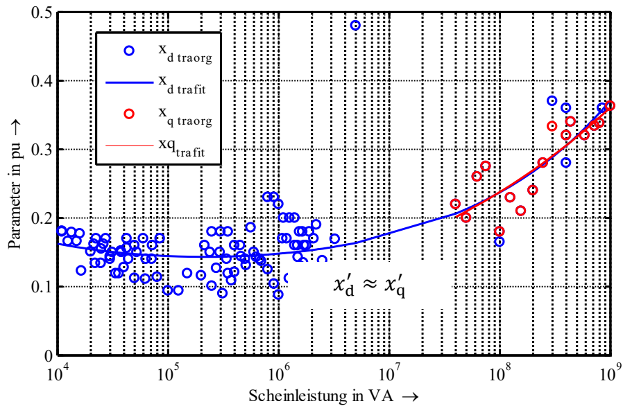
Abbildung 101: Transiente Reaktanzen der d- und q-Achse in Abhängigkeit von der Bemessungscheinleistung (Punkte: originale Beispieldaten; Linie: approximierte Annahme)
