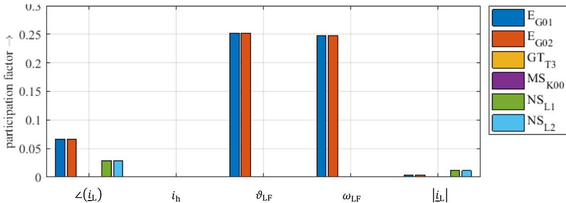
Abbildung 74: Auswirkung der Modellordnung (blau=sub-konst-RL, grün=sub-konst-RLq, türkis=tra-konst-RLq, rot=tram-konst-RLq und orange=sta-konst-RLq) auf die Eigenwerte im Höchstspannungsnetz (NS) bei der Annahme von konstanten Quellenspannungen
