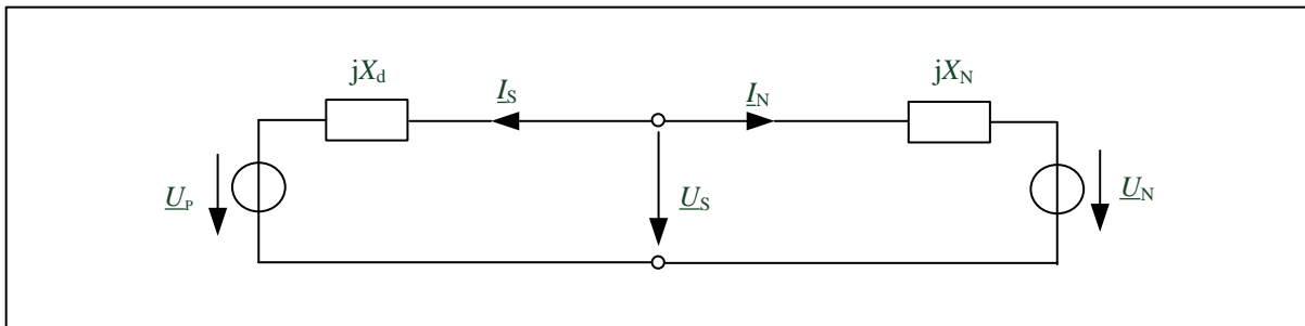
Abbildung 10: Elektrisches Ersatzschaltbild der Einmaschinenanordnung für stationäre Berechnungen
