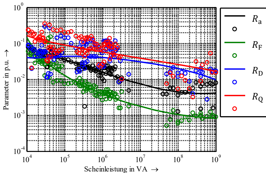
Abbildung 34: Bezogene Ständer- und Läuferwiderstände in Abhängigkeit von der Bemessungsscheinleistung (Punkte: originale Beispieldaten; Linie: angenäherte Annahme)
