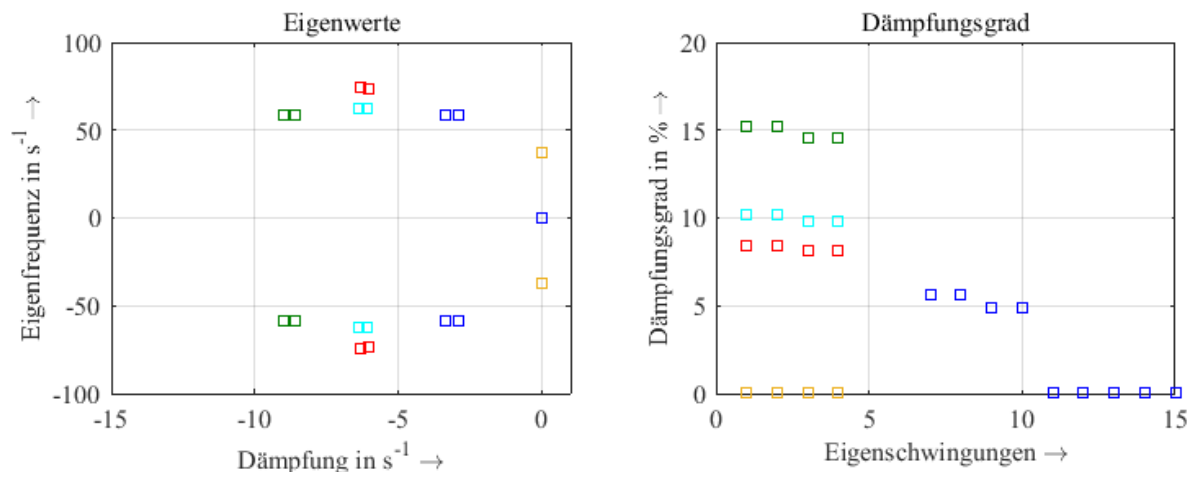
Partizipation an den Eigenwerten 9 und 10 ( -3 \pm j59 ) s^{-1} , für sub-konst-RL mit Dämpfungsgrad von 4,9 %
