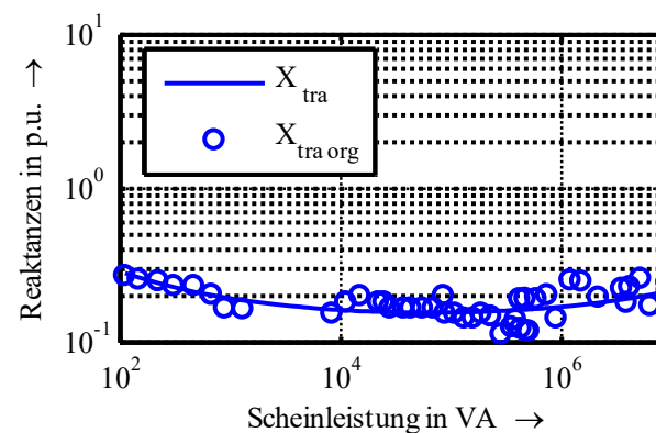
Abbildung 40: Transiente Reaktanz in Abhängigkeit von der Bemessungsscheinleistung (Punkte: originale Beispieldaten; Linie: approximierte Annahme)
