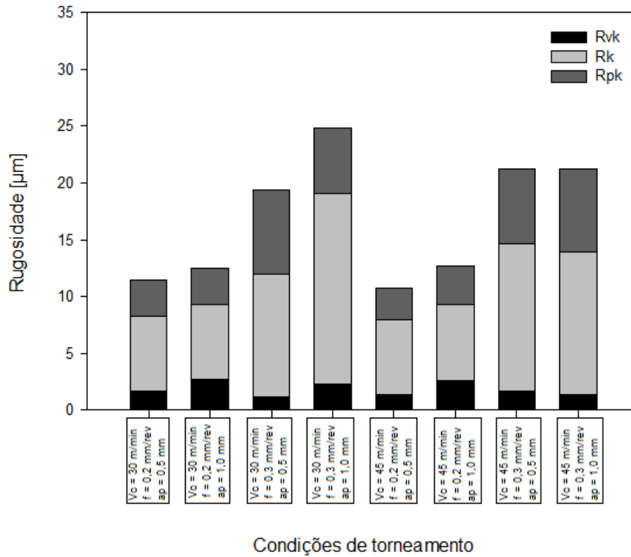
Figura 8: Variação da profundidade de vales reduzida (Rvk), profundidade da rugosidade central (Rk) e altura de pico reduzida (Rpk) com os parâmetros de corte.
