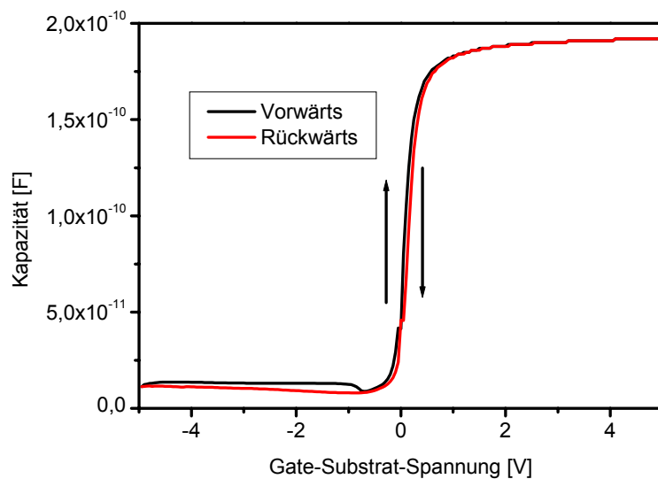
Abb. 62 HF-C(U)-Hysterese-Messung an einem Al-MOS-Kondensator mit einer 11 nm dicken BTBAS-SiO 2 -Schicht. Die sehr geringe Hysterese macht deutlich, dass in diesem Isolator nur sehr wenig Ladung gespeichert wird. (Prozessparameter: T = 500°C, p = 200 mTorr, BTBAS = 20 sccm, O 2 /N 2 = 80 sccm, Messbedingung: Padgröße: 6,25 \times 10^{-4} \text{ cm}^2 , HF: 100 kHz, NF: quasistatisch, Integrationszeit: 0,1 s)
