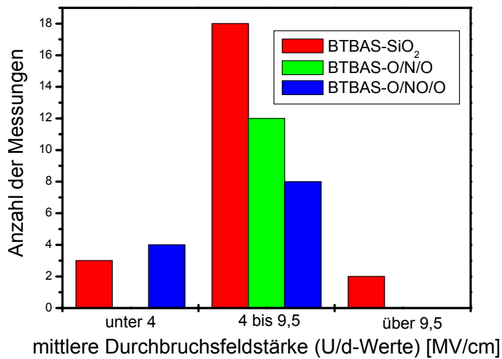
Abb. 72 Darstellung der mittleren Durchbruchfeldstärke-Verteilung (U/d-Werte) von BTBAS-SiO 2 -, -O/N/O- und -O/NO/O-Proben (Padgröße: 6,25x10 -4 cm 2 )
