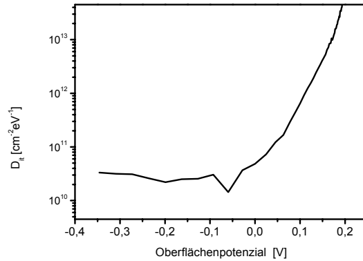
Abb. 59 Grenzflächenzustandsdichte einer BTBAS-SiO 2 ermittelt aus der HF- und NF-C(U)-Messung dargestellt in Abb. 58
