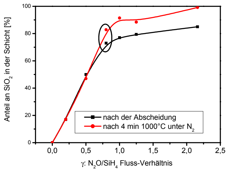
Abb. 96 Auswirkung des Gasverhältnisses N_2O/SiH_4 auf den Anteil an SiO_2 in der Schicht vor und nach der Temperung. Das Verhältnis kann kontinuierlich zwischen reinem Silizium und reinem SiO_2 eingestellt werden. Eine Begrenzung ist hier nur durch die MFCs der Anlage gegeben, wodurch das Verhältnis \gamma auf 2,25 limitiert ist (weitere Prozessparameter: T = 600\text{ °C} , p = 200\text{ mTorr} - als Standardparameter wurde \gamma = 0,8 gewählt und durch einen Kreis in dieser Grafik markiert).
