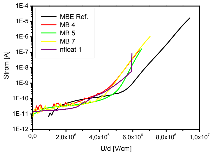
Abb. 115 Typische Strom-/Spannungskennlinie von n^+ -Poly-Si-MOS-Kondensatoren mit SIPOS-, BTBAS- und n^+ -Poly-Si-Speicherschichten im Vergleich zu einer Referenzprobe ohne Nano-Cluster: Referenzprobe: MBE Ref., SIPOS: MB 5, BTBAS: MB 4 und 7, n-Polysilizium: nfloat 1 (Messbedingungen: Spannungsrampe: aufsteigend, n-Substrat: positive Spannung am Gate, Padgröße: 6,25 \times 10^{-4} \text{ cm}^2 , Integrationszeit: 0,8 s)
