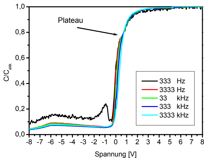
Abb. 71 Frequenzabhängige C(U) -Messung an einem n^+ -Poly-Si-MOS-Kondensator mit einer BTBAS-O/NO/O-Schicht als Isolator. Die C(U) -Messung weist im Anstieg zur Akkumulationskapazität ein Plateau auf, welches mit zunehmender Messfrequenz schwächer ausgeprägt ist. (Messbedingung: Padgröße: 6,25 \times 10^{-4} \text{ cm}^2 , HF: 333 Hz, 3333 Hz, 33 kHz, 333 kHz, 3333 kHz, Spannungsrampe: abfallend, Integrationszeit: 0,1 s. Als C_{\text{akk}} wurde aus jeder Messung die höchste HF-Kapazität benutzt.)
