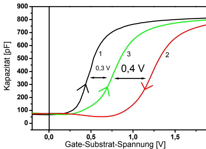
Abb. 118 HF-C(U)-Messung an einem n + -Poly-MOS-Kondensator mit Silizium-Nano-Clustern (MBE 6): 1) Ausgangsmessung im unprogrammierten Zustand, 2) Messung nach einer Programmierung (~ Sekunden) bei +12 V, 3) Messung nach einer Löschung (~ Sekunden) bei -12 V (Messbedingung: Padgröße: 6,25 \times 10^{-4} \text{ cm}^2 , HF: 100 kHz, Integrationszeit: 0,1 s, Spannungsbereich Messung 1-3 : -1,5 V - 2 V)
