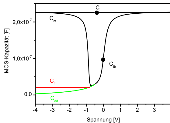
Abb. 39 Darstellung einer C(U) -Messung an einer MOS-Struktur über der Biasspannung. Die Unterschiede bei niedriger ( C_{nf} ), hoher ( C_{hf} ) Messfrequenz sowie sehr schneller Biasänderung ( C_{dd} ) wurden herausgestellt.
