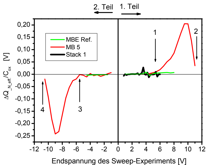
Abb. 133 Auswertung des Sweep-Experiment mit MOS-Kondensatoren mit Silizium-Nano-Clustern (SIPOS-Abscheidung, Proben: Stack 1 und MB 5): \Delta Q_{N,eff.} stellt für jeden Messzyklus während des Sweep-Experiments die effektiv programmierte bzw. gelöschte Ladung dar. Im ersten Teil des Experiments sind deutlich Beladungspeaks zu erkennen: 1 Beginn der Programmierung, 2 Ende der Programmierung. Im zweiten Teil treten bei der Löschung diese Peaks genauso deutlich auf, 3 Beginn der Löschung, 4 Ende der Löschung.
