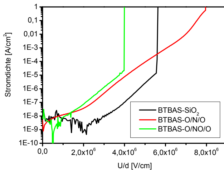
Abb. 73 Darstellung der Stromdichte in Abhängigkeit der mittleren Feldstärke (U/d-Werte) eines MOS-Kondensators mit einer BTBAS-SiO 2 -, -O/N/O- und -O/NO/O-Schicht als Isolator (Padgröße: 6,25x10 -4 cm 2 , als Schichtdicken wurden die SE-Ergebnisse herangezogen)
