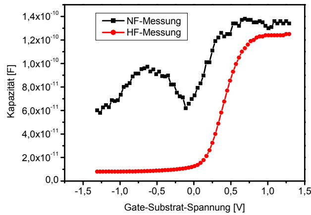
Abb. 69 HF- und NF-C(U)-Messung an einem n + -Poly-Si-MOS-Kondensator mit einer O/NO/O-Schicht als Isolator (Messbedingung: Padgröße: 6,25x10 -4 cm 2 , HF: 100 kHz, NF: quasistatisch, Spannungsrampe: abfallend, Integrationszeit: 0,1 s)
