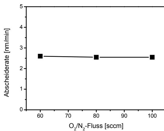
Abb. 53 Darstellung der nach Taguchi berechneten Abscheiderate von BTBAS-SiO 2 über dem O 2 /N 2 -Fluss während des Prozesses (Verbindung zwischen den Messpunkten stellt nur eine Hilfslinie dar)
