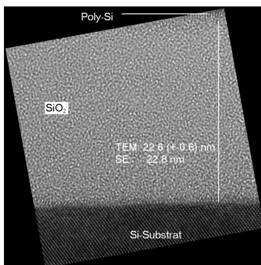
Abb. 108 Hochauflöste cross-section TEM-Messung an der Probe Imp 12_2_T2: Die ermittelte Isolator-Schichtdicke liegt bei 22,6 nm ±0,6 nm. Der Fehler resultiert aus der Annahme, dass bei der graphischen Auswertung der TEM-Messung eine Unsicherheit von 2,5 % vorliegt. Im Vergleich dazu wurde unabhängig mittels SE eine Schichtdicke von 22,8 nm bestimmt.
