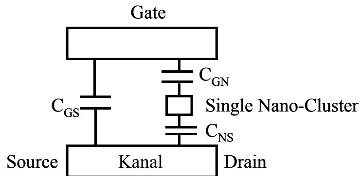
Abb. 19 Kapazitives Ersatzschaltbild eines Einzelektronen-Speichers
