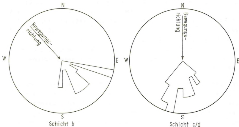
Abb.1 : Geschiebeeinregelung
